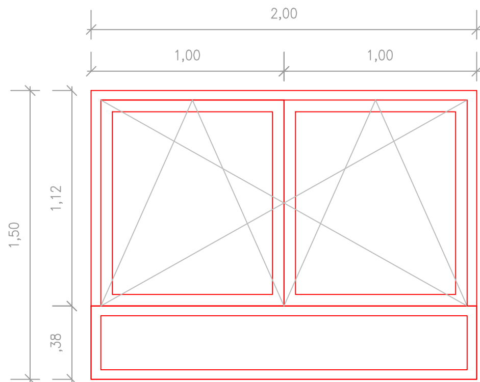
C-1: 14 uds. VENTANA OSCIOBATIENTE DE PVC DE DOS HOJAS CON MONTANTE INFERIOR FIJO
