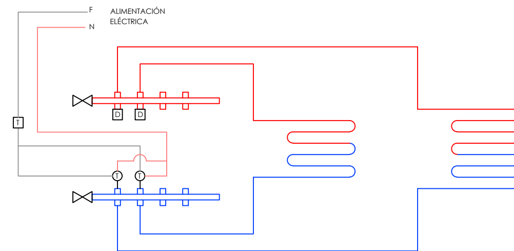
ESQUEMA CONTROL DE TEMPERATURA TERMOSTATO ELÉCTRICO CONVENCIONAL.
