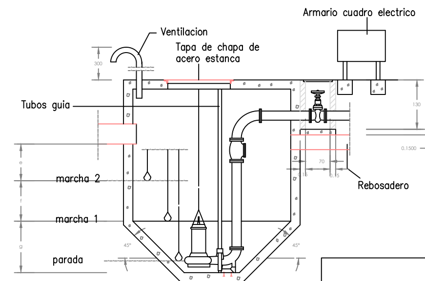
Seccion A-A
