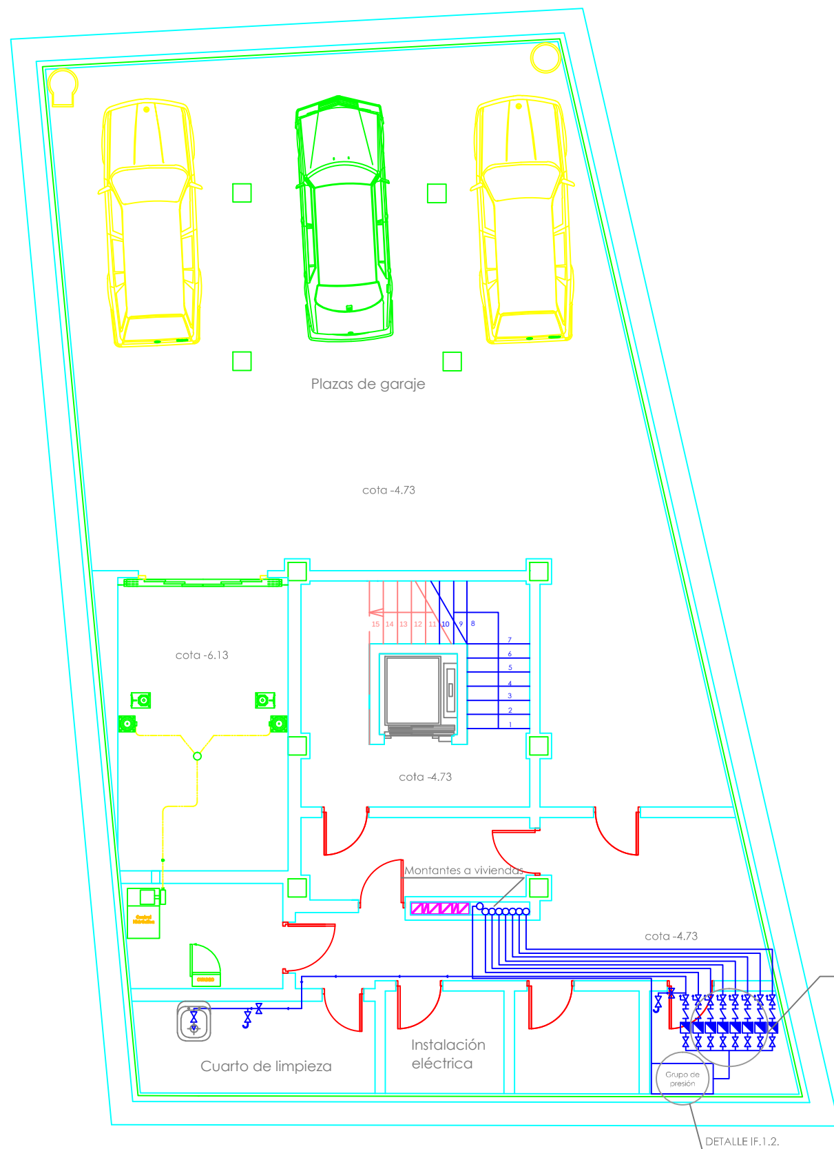
Planta Sótano 2º
