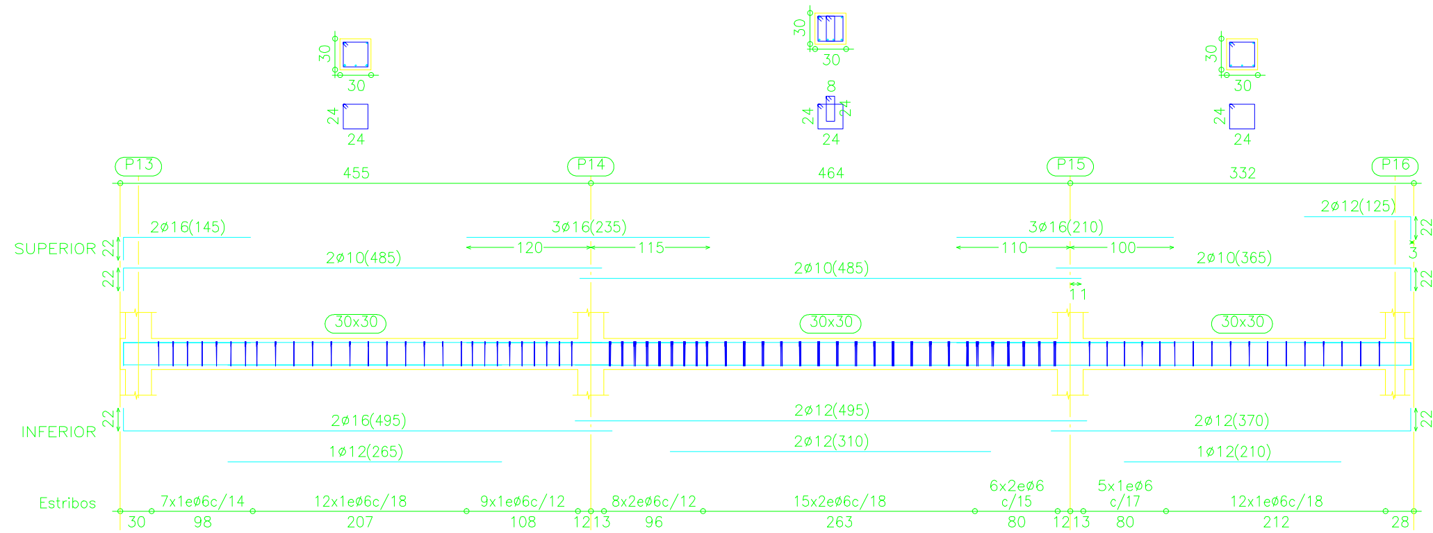
Pórtico 9
