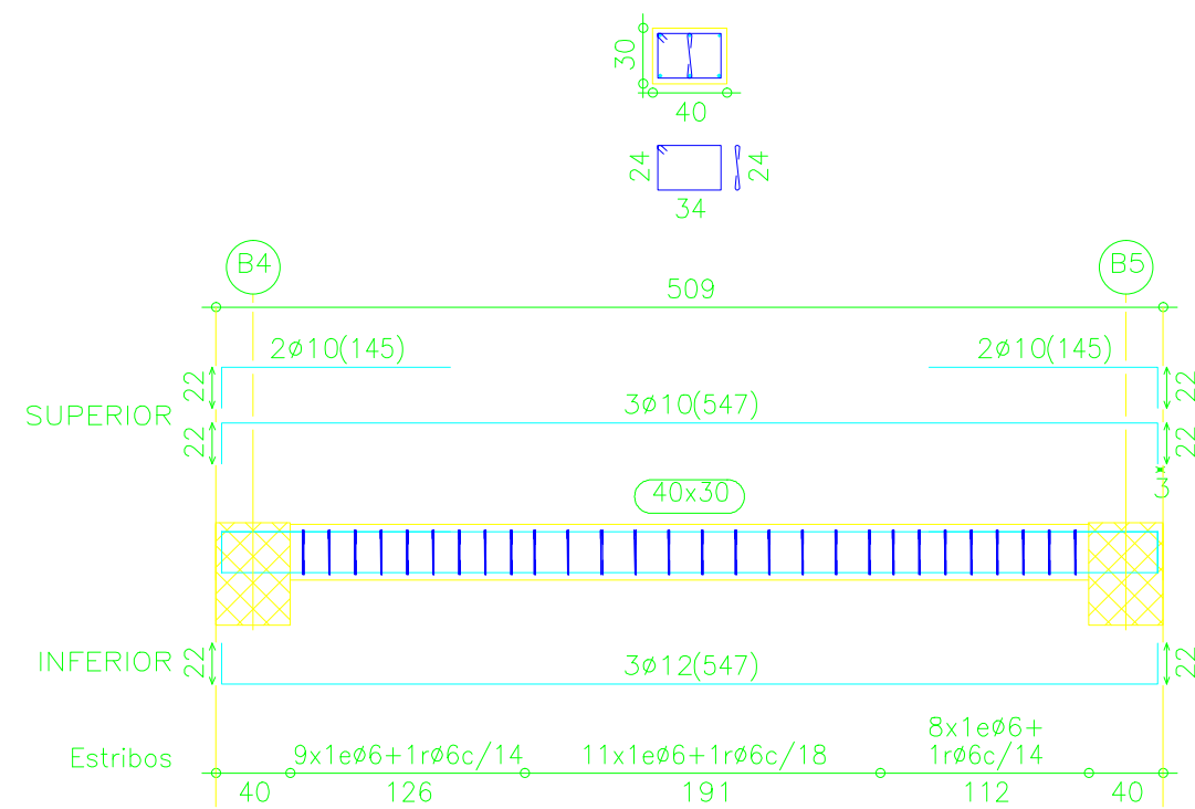
Pórtico 1
