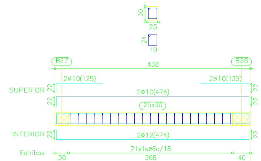
Pórtico 16
