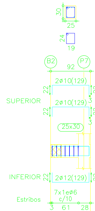
Pórtico 15
