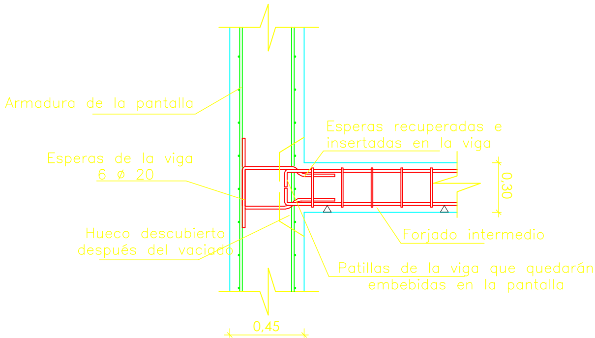
Detalle 6: Encuentro de viga intermedia con pantalla
