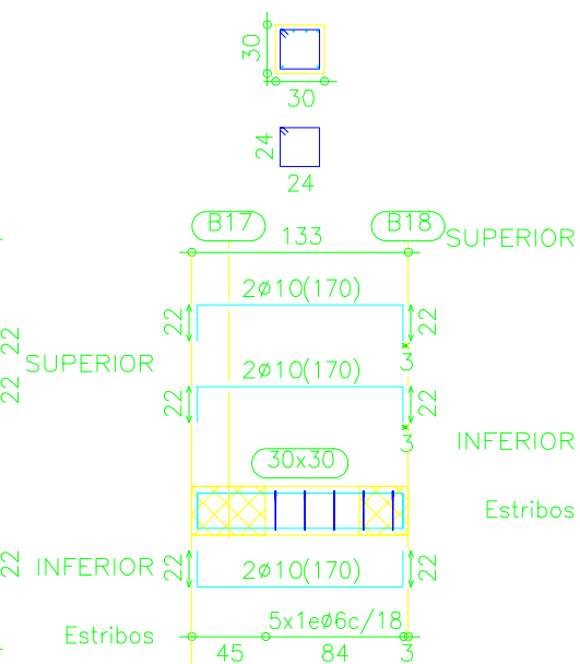
Pórtico 10
