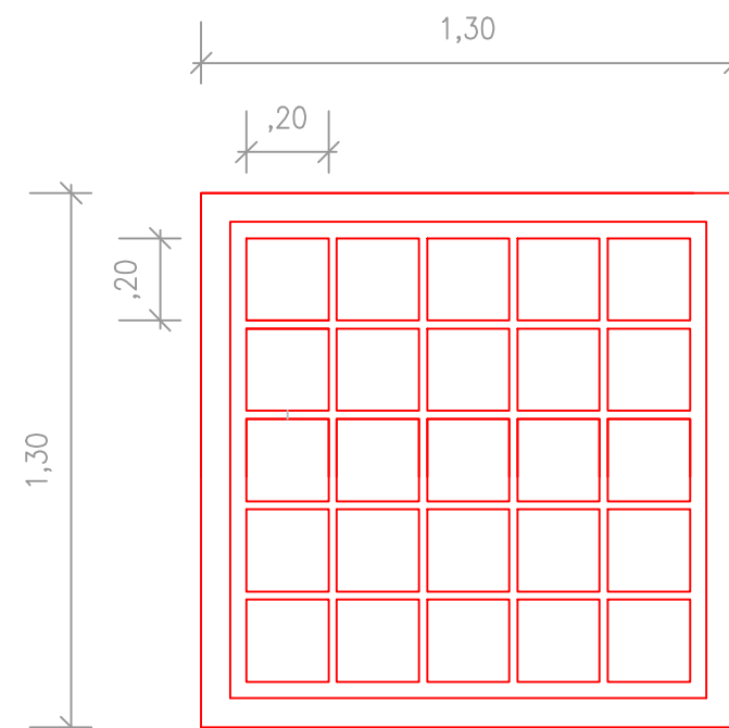
C-8: 1ud. HUECO DE VIDRIO MOLDEADO,PIEZAS 20X20X8
