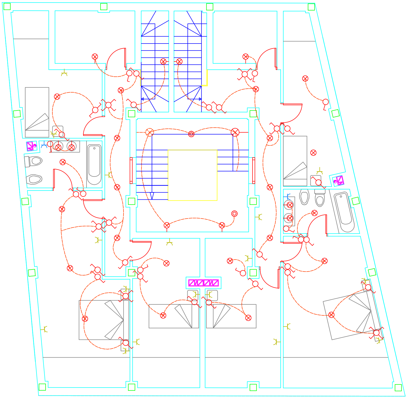
PLANTA 2º DE DÚPLEX
