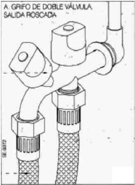
DETALLE IF.3.2.
