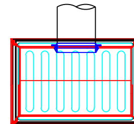
ARQUETA SUMIDERO SIFÓNICA DE POLIPROPILENO REFORZADO 58X35X60 E: 1/20
