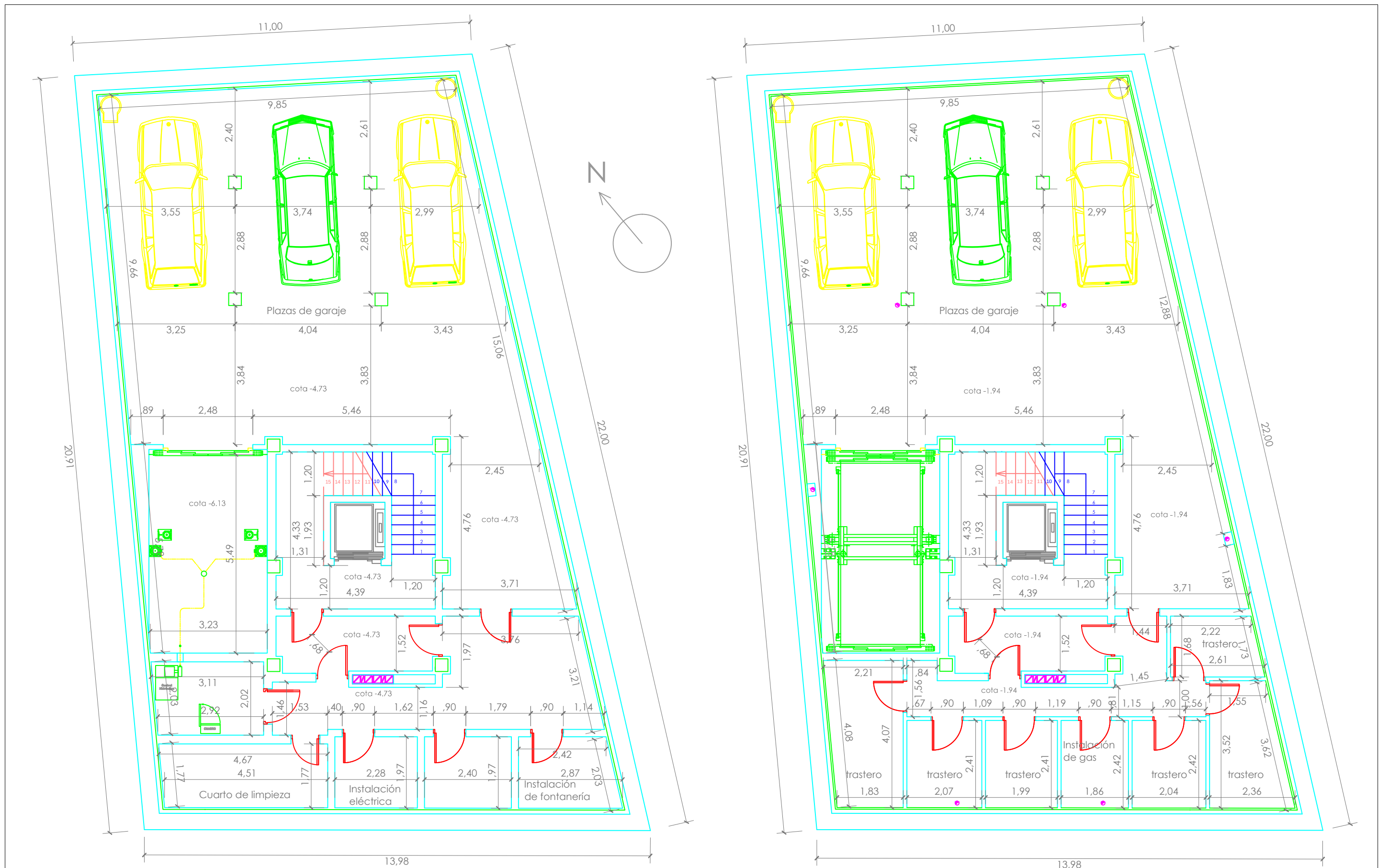
Planta Sótano 2º
