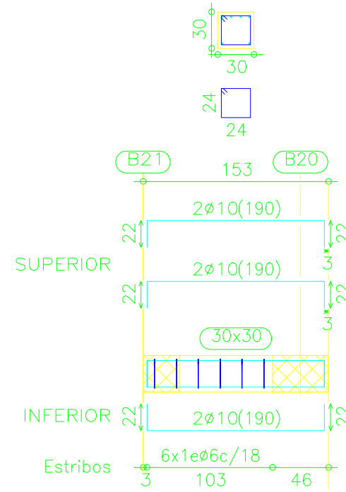
Pórtico 8
