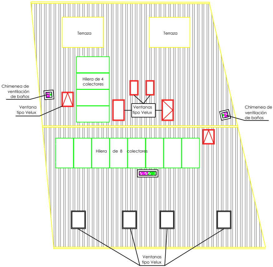
Planta de cubierta con la disposición de los colectores solares
