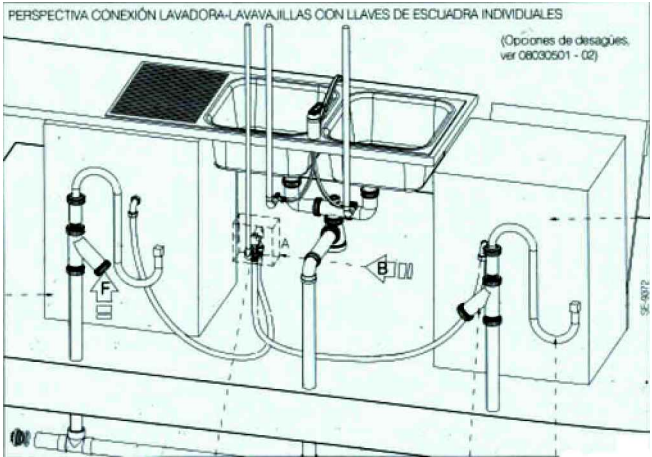
DETALLE IF.3.1.
