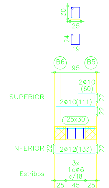
Pórtico 17
