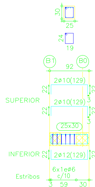
Pórtico 14
