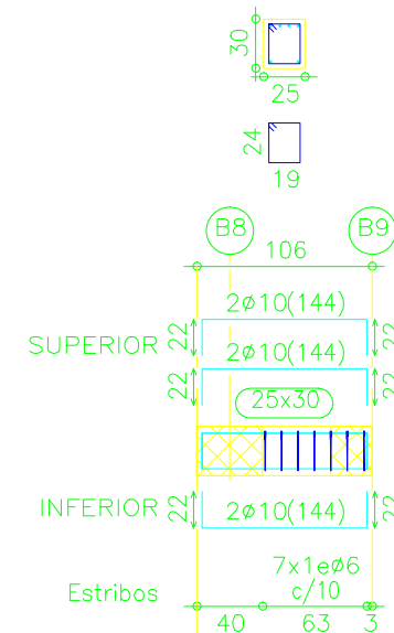
Pórtico 10
