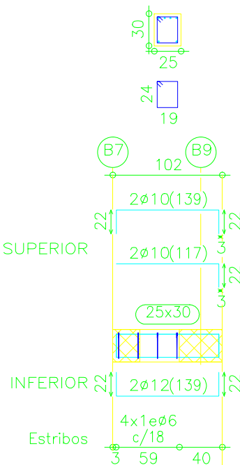
Pórtico 16
