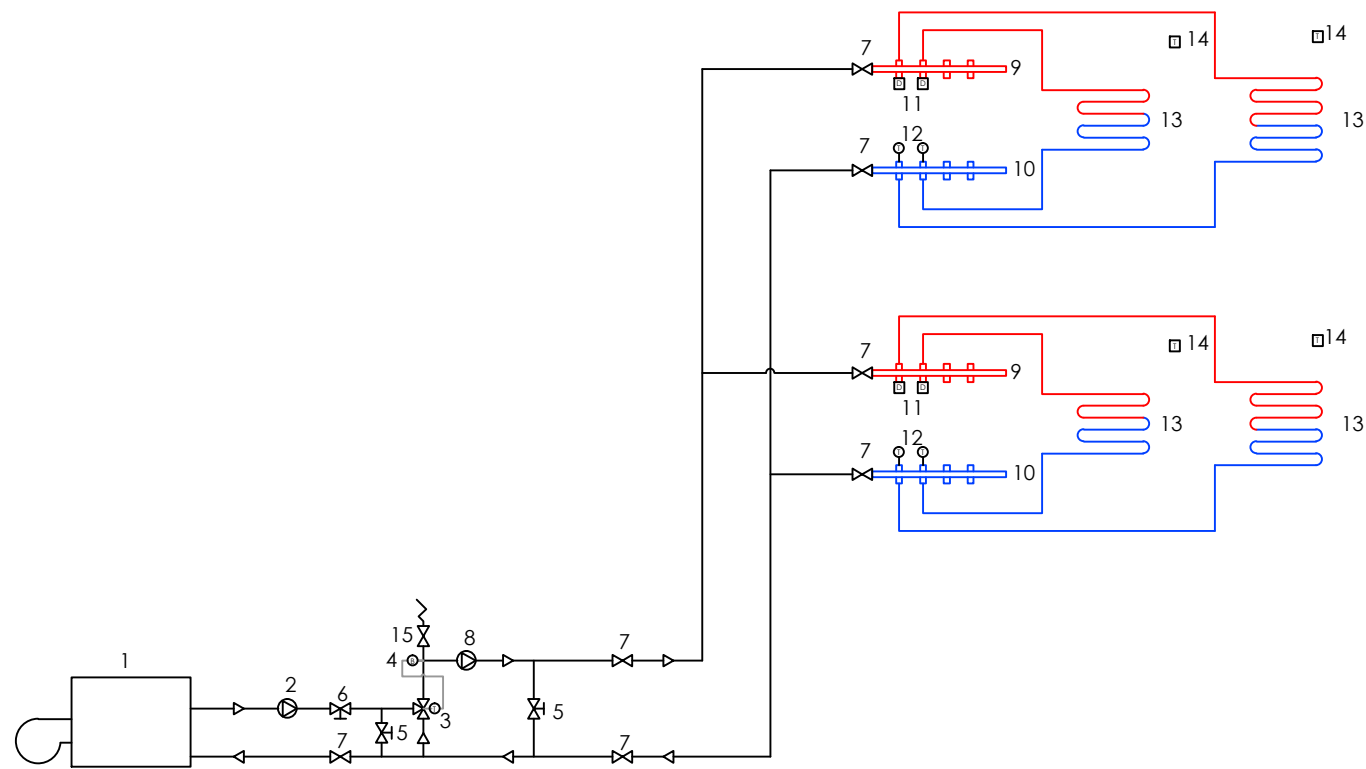
ESQUEMA CIRCUITO PLANTA DÚPLEX
