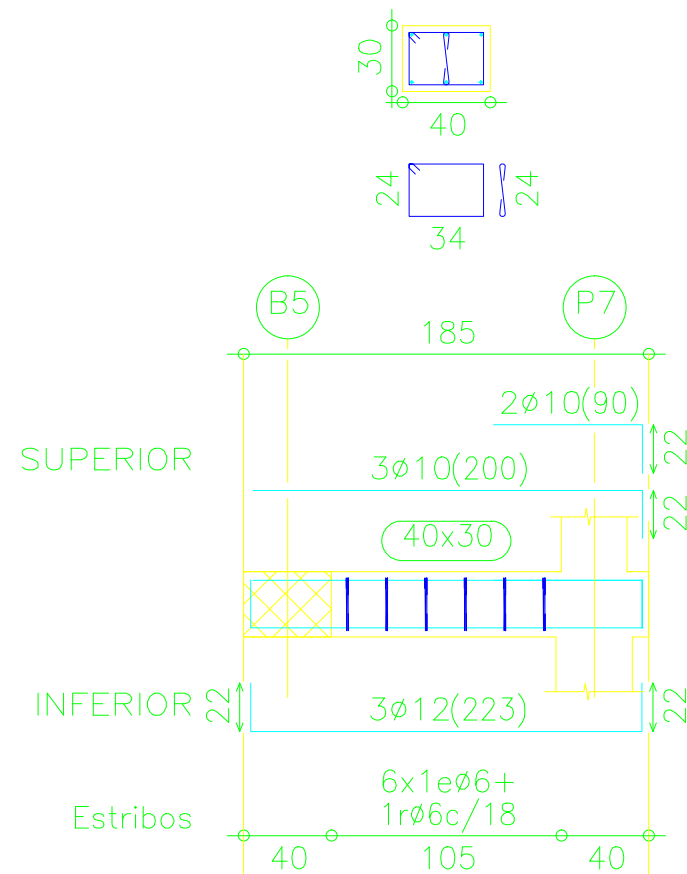
Pórtico 20
