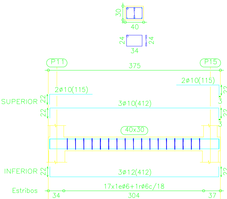
Pórtico 18
