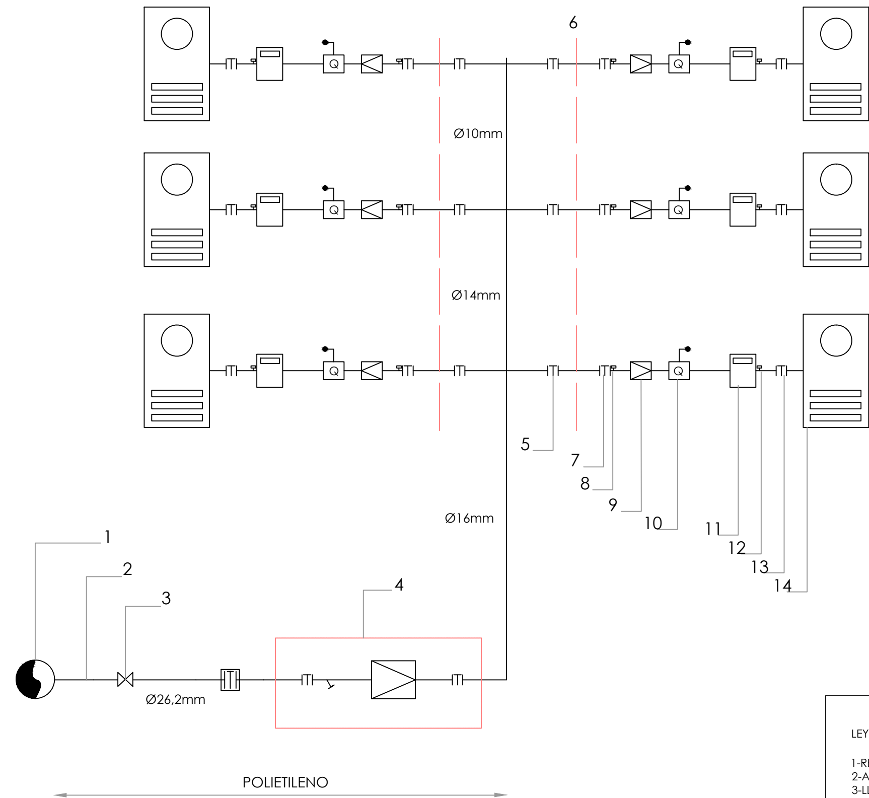
ESQUEMA DE INSTALACIÓN CONTADORES EN VIVIENDA
