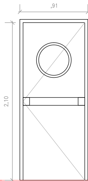
C.I-2: 8 uds. PUERTA VESTÍBULOS INDEPENDENCIA METÁLICA PRACTICABLE 1 HOJA, RESISTENTE AL FUEGO 60 minutos, HOMOLOGADA ANTES "RF60" Y CON CODIGO TECNICO "EI 2 60-C5"
