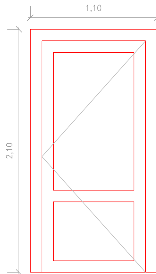
C-7: 1ud. PUERTA DE PATIO DE ALUMINIO Y CRISTAL DE SEGURIDAD, DE UNA HOJA
