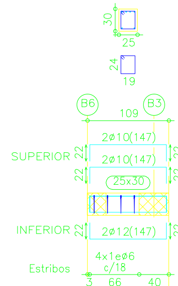
Pórtico 8
