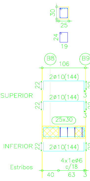
Pórtico 8
