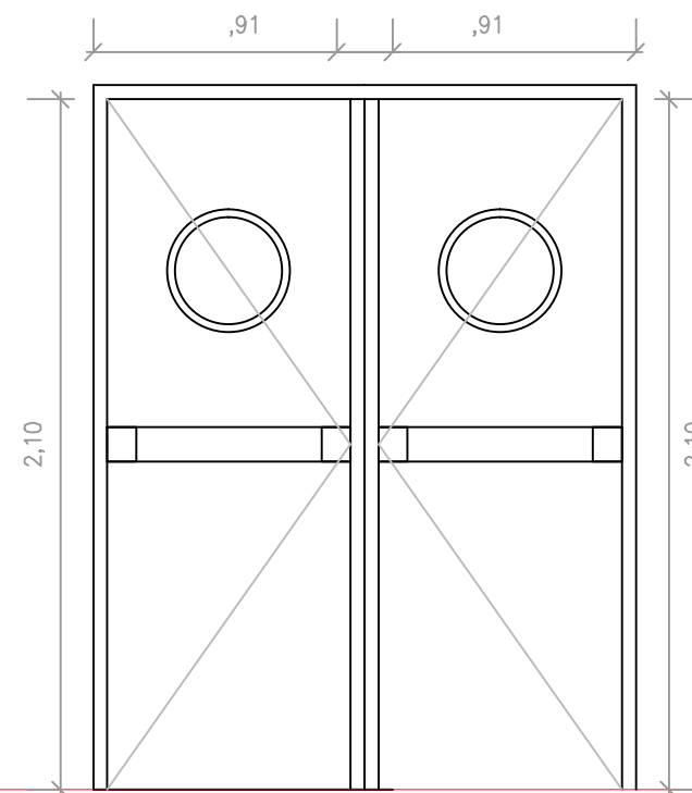
C.I-3: 3 uds. PUERTA VESTÍBULOS INDEPENDENCIA METÁLICA PRACTICABLE 2 HOJAS, RESISTENTE AL FUEGO 60 minutos, HOMOLOGADA ANTES "RF60" Y CON CODIGO TECNICO "EI 2 60-C5"
