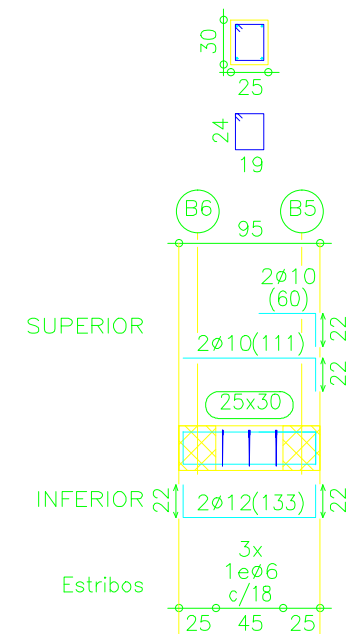
Pórtico 17
