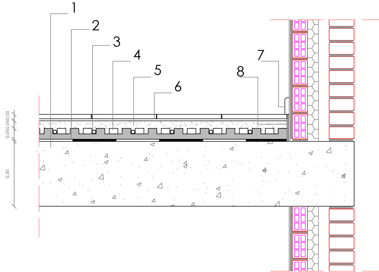
SECCIÓN CONSTRUCTIVA PAVIMENTO CERÁMICO/PARQUET E:1/10
