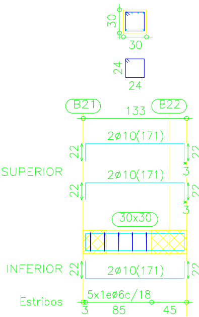
Pórtico 17
