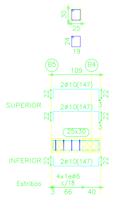
Pórtico 5
