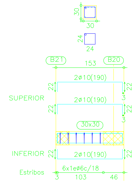
Pórtico 11
