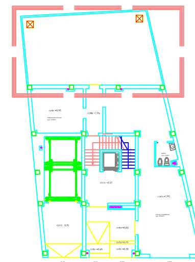
PLANTA BAJA
