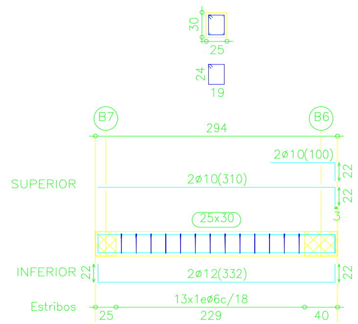
Pórtico 2
