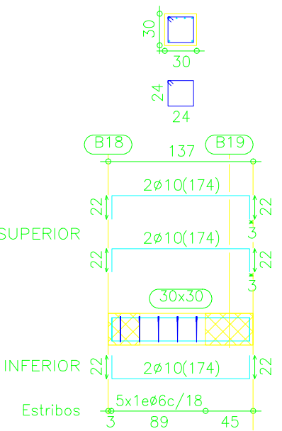
Pórtico 12
