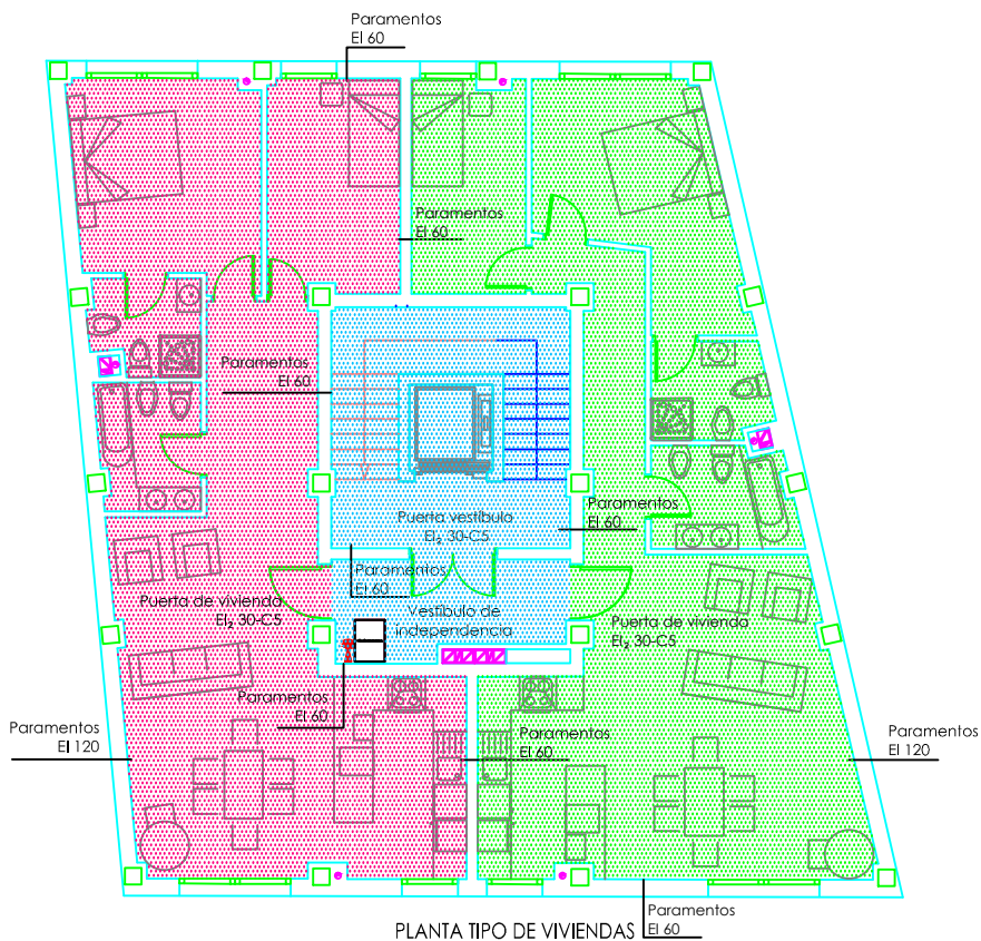
PLANTA TIPO DE VIVIENDAS
