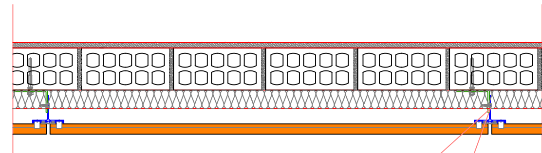
SECCIÓN HORIZONTAL E: 1/10
