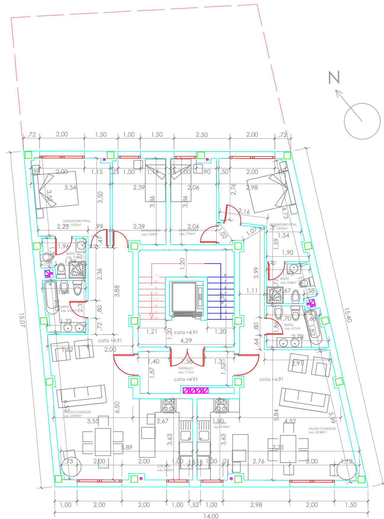
Planta Primera y Segunda
