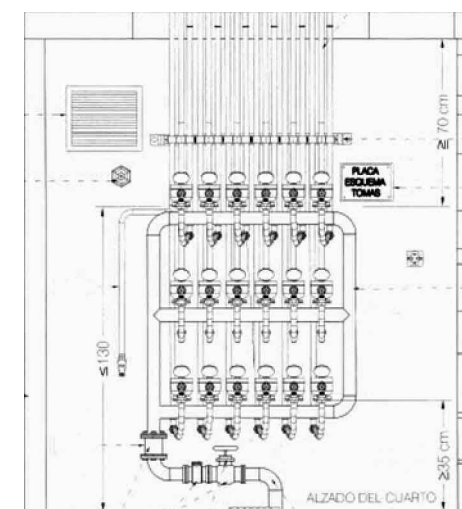
DETALLE IF.1.1. ALZADO DE CONTADORES
