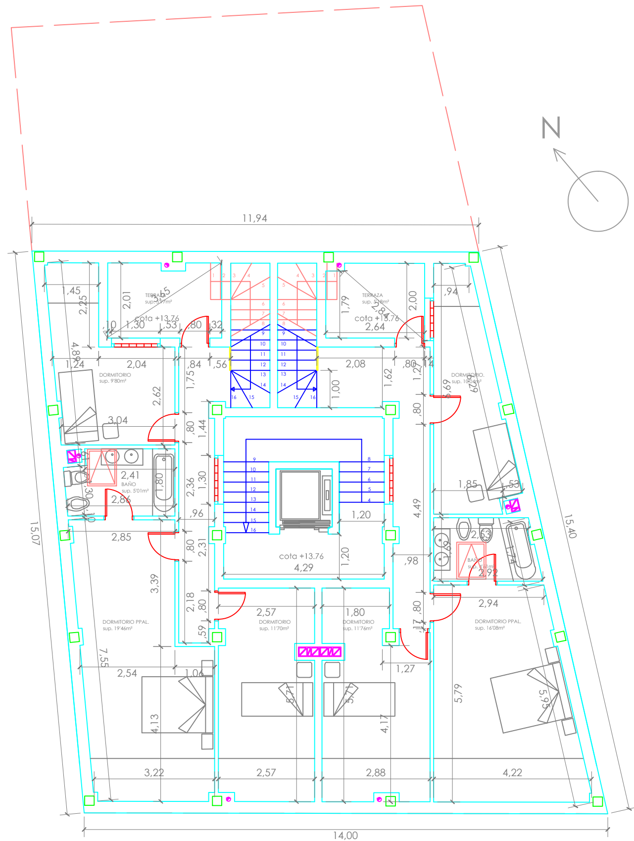
Planta Bajo cubierta 2º Nivel Dúplex
