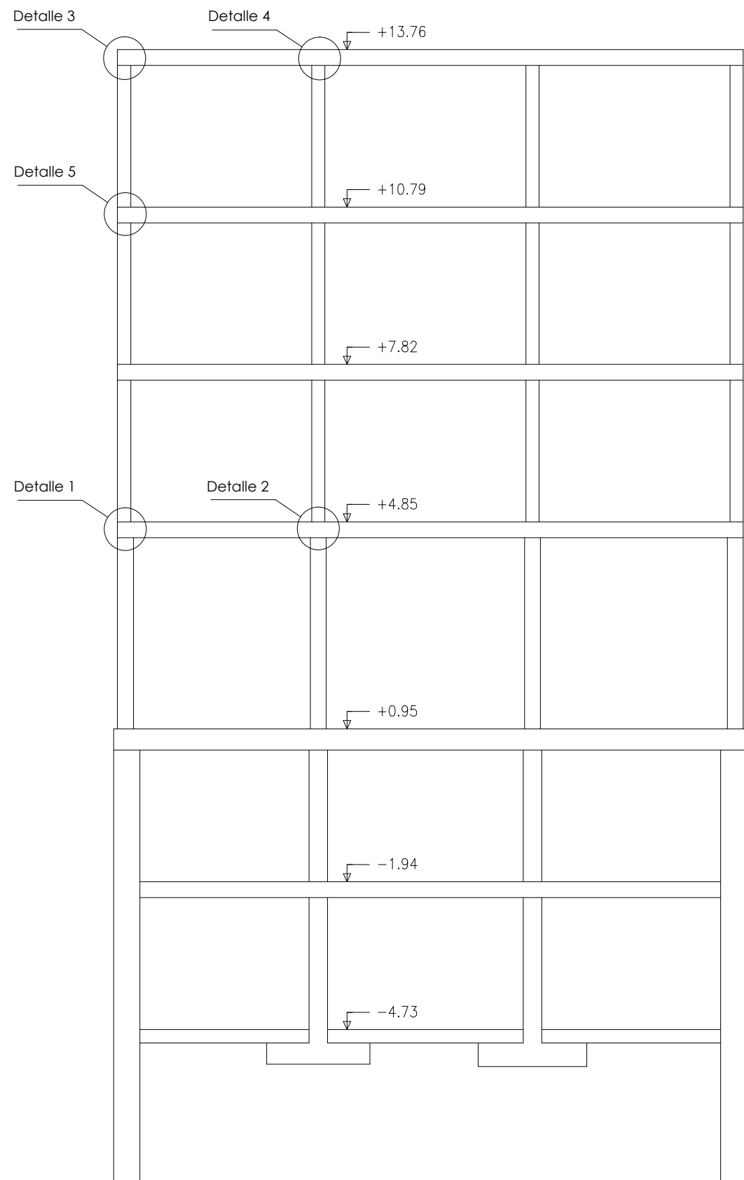
ALINEACIÓN 5
