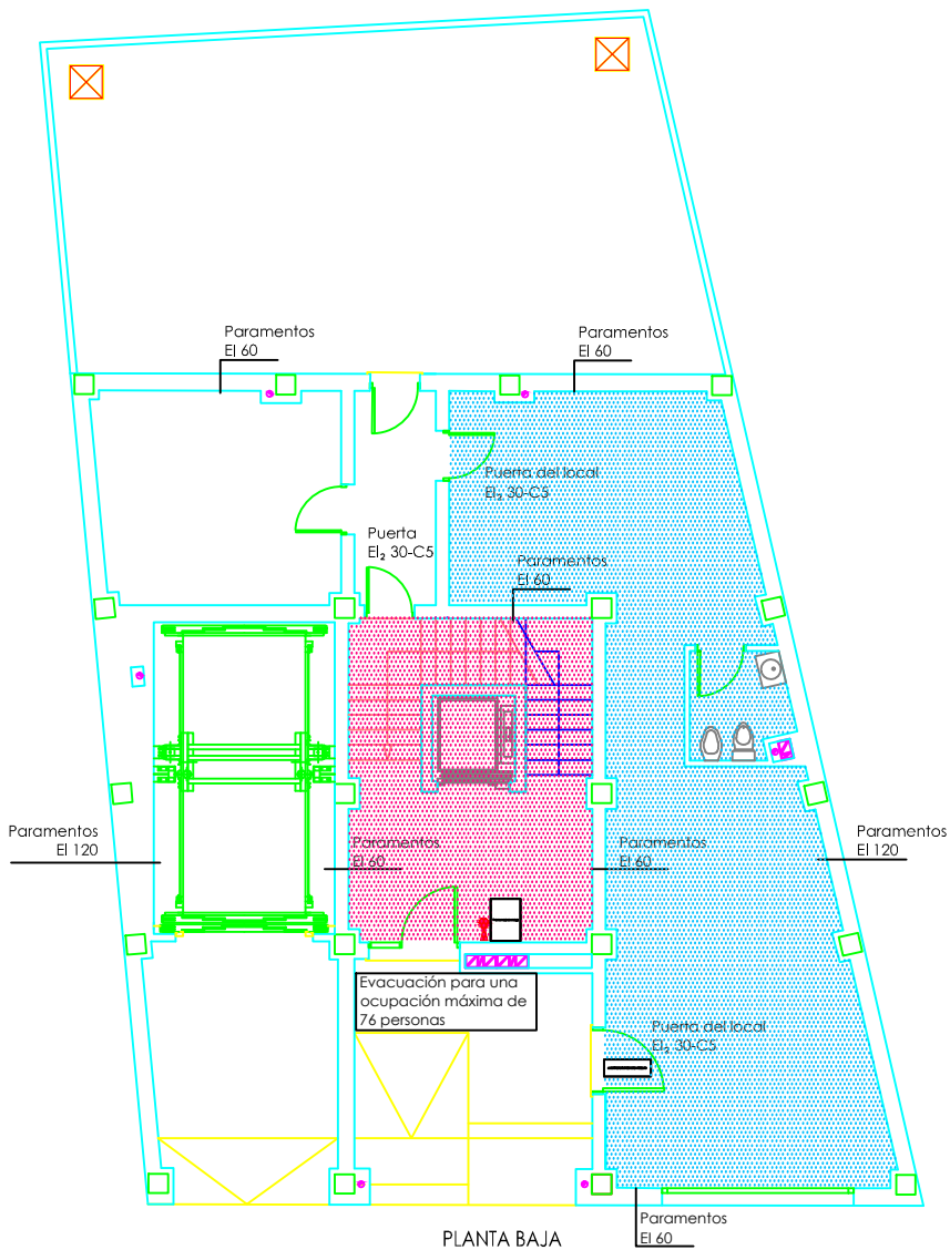
PLANTA BAJA
