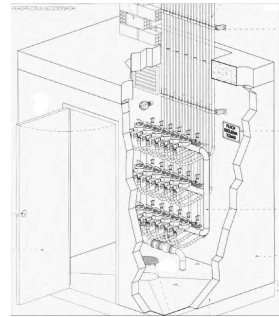
DETALLE IF.6.2. Perspectiva seccionada del cuarto de contadores.
