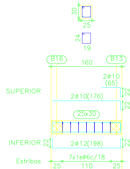
Pórtico 4
