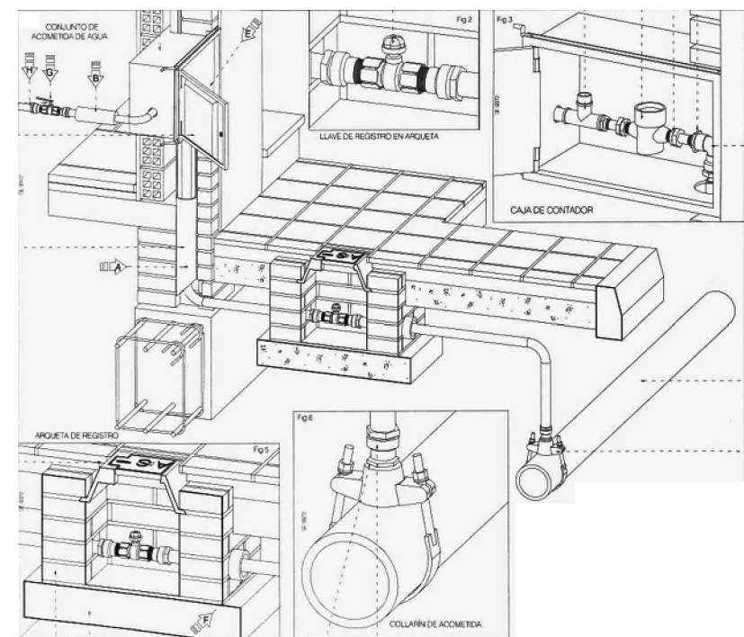
DETALLE IF.6.1. Collarín de acometida con llave de toma desde red de distribución. Arqueta de registro con llave de registro general. Caja de contador junto con el resto de elementos de acometida.
