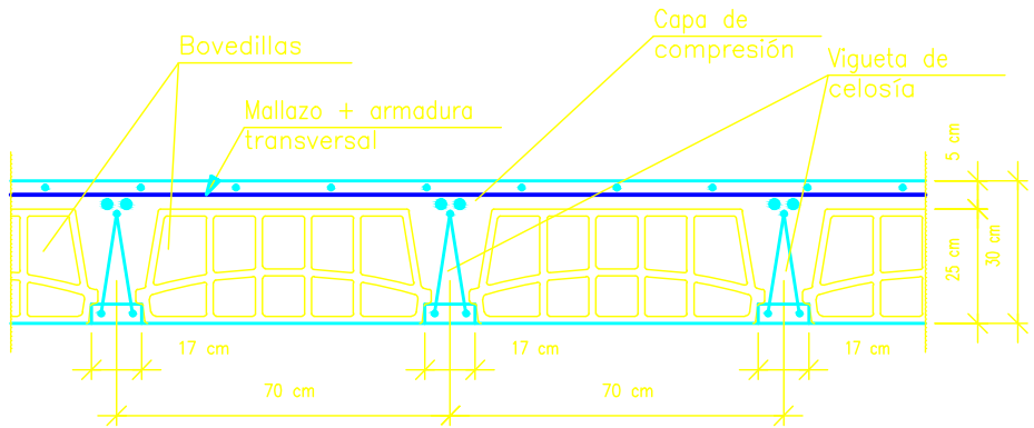
Sección de forjado unidireccional de viguetas de celosía
