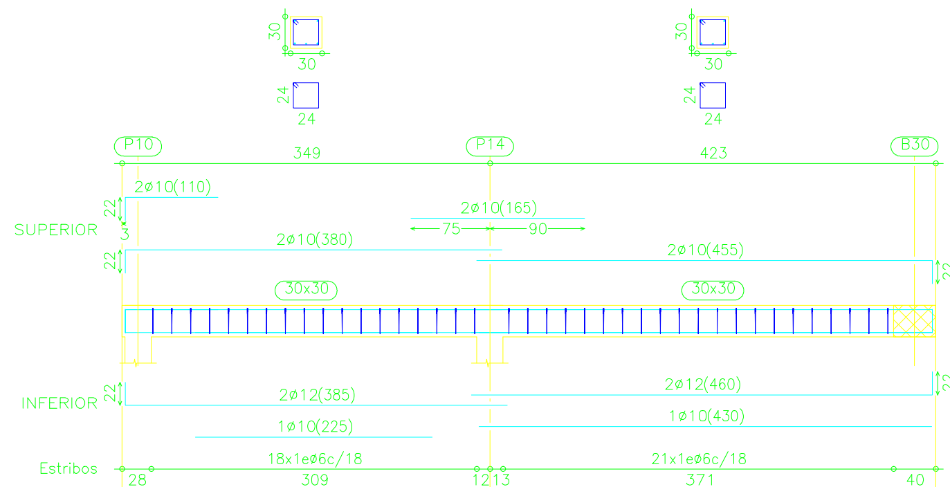
Pórtico 15
