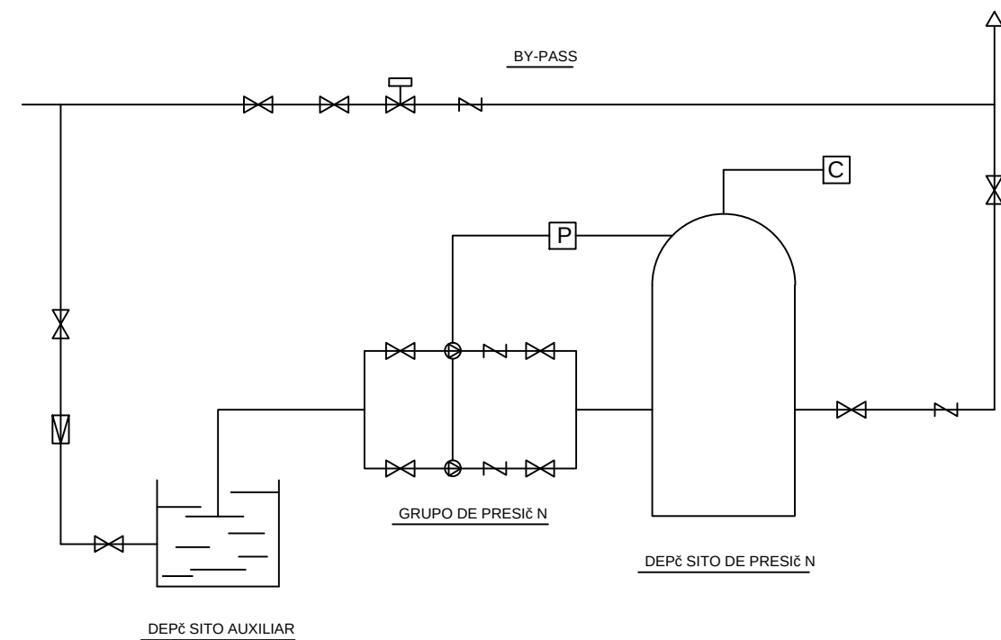
DETALLE IF.1.2.
