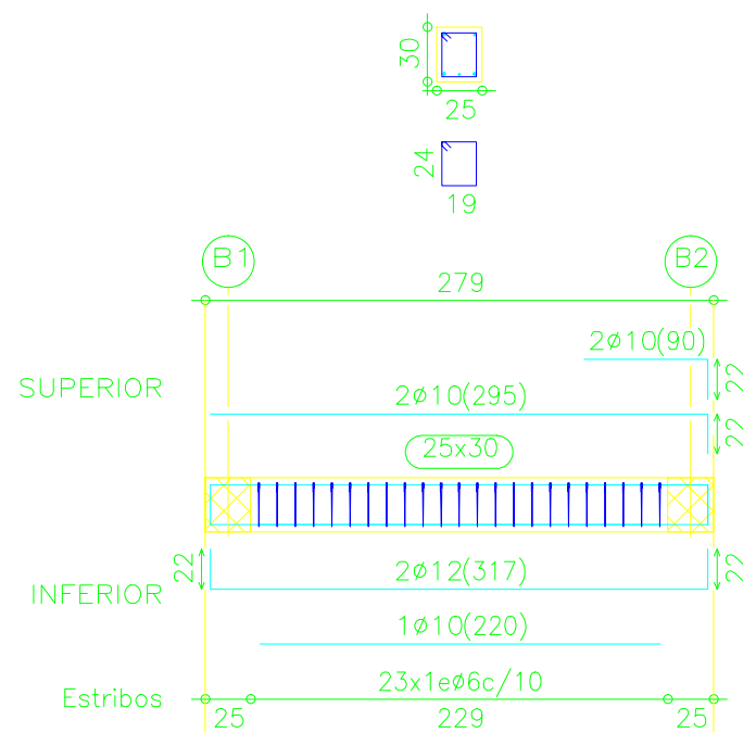
Pórtico 2
