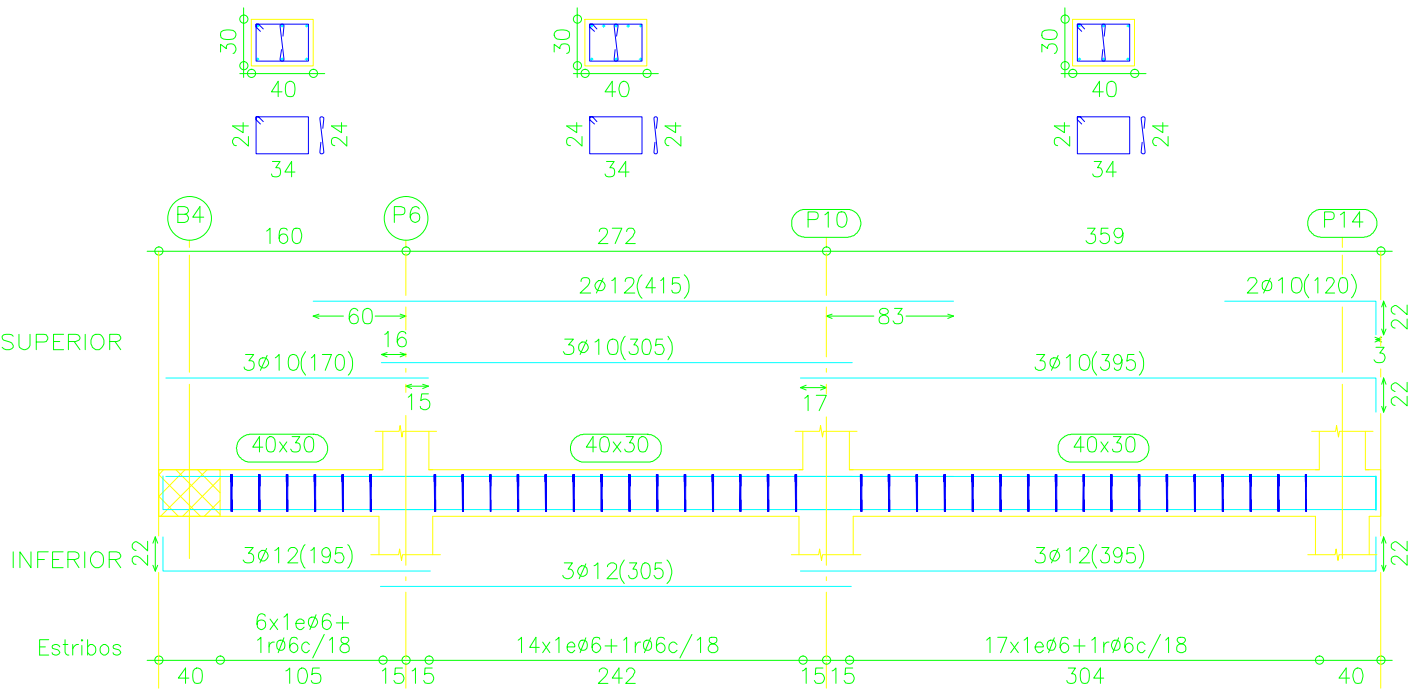
Pórtico 14
