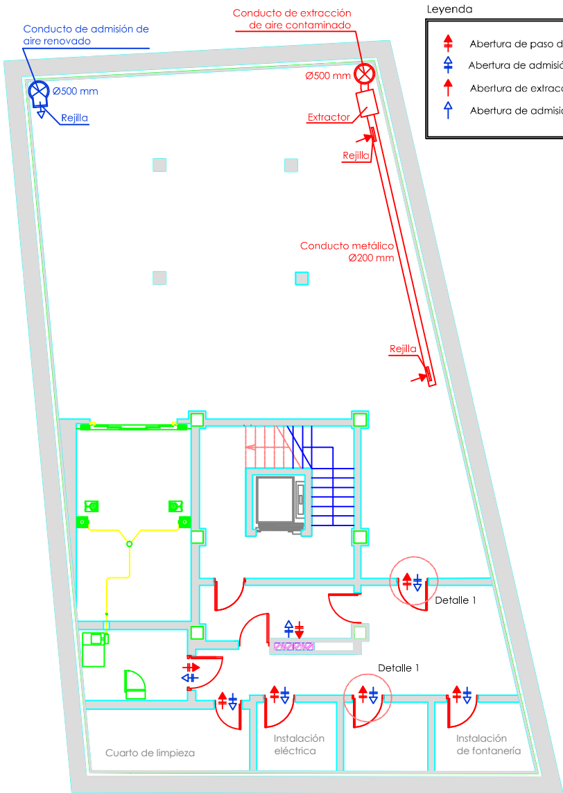
PLANTA SÓTANO 2
