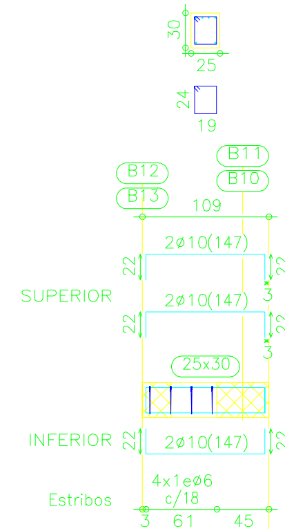
Pórtico 5 Pórtico 6
