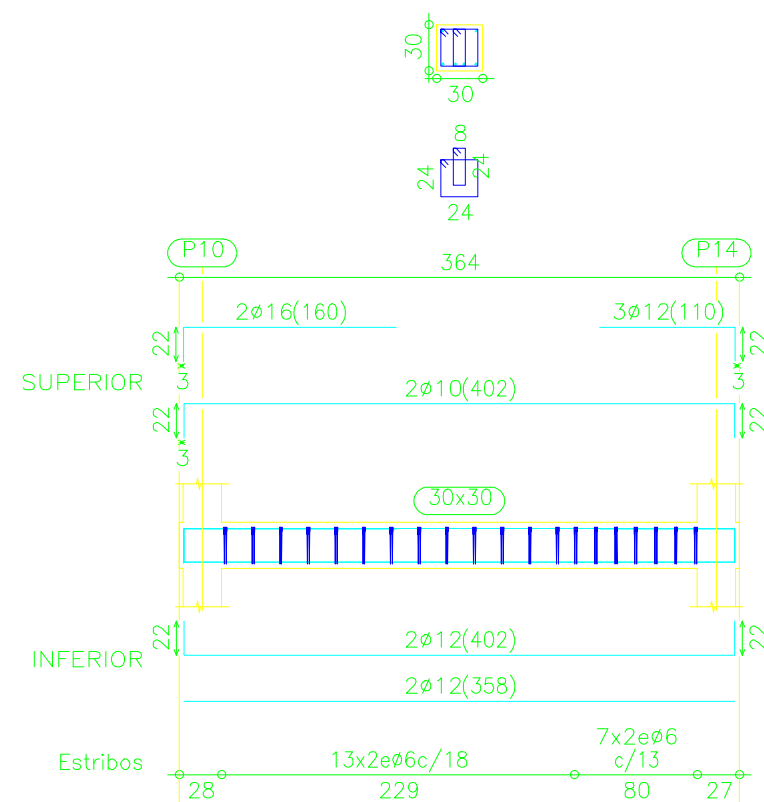
Pórtico 13
