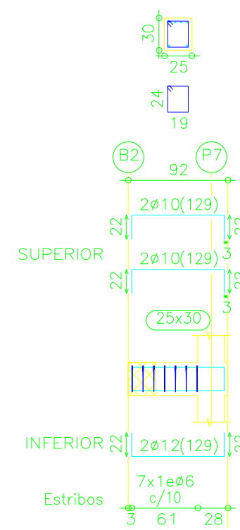
Pórtico 15
