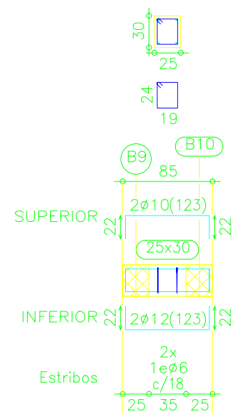
Pórtico 14
