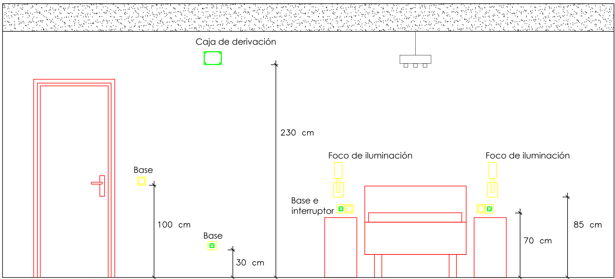
Dotación eléctrica acotada tipo de los dormitorios
