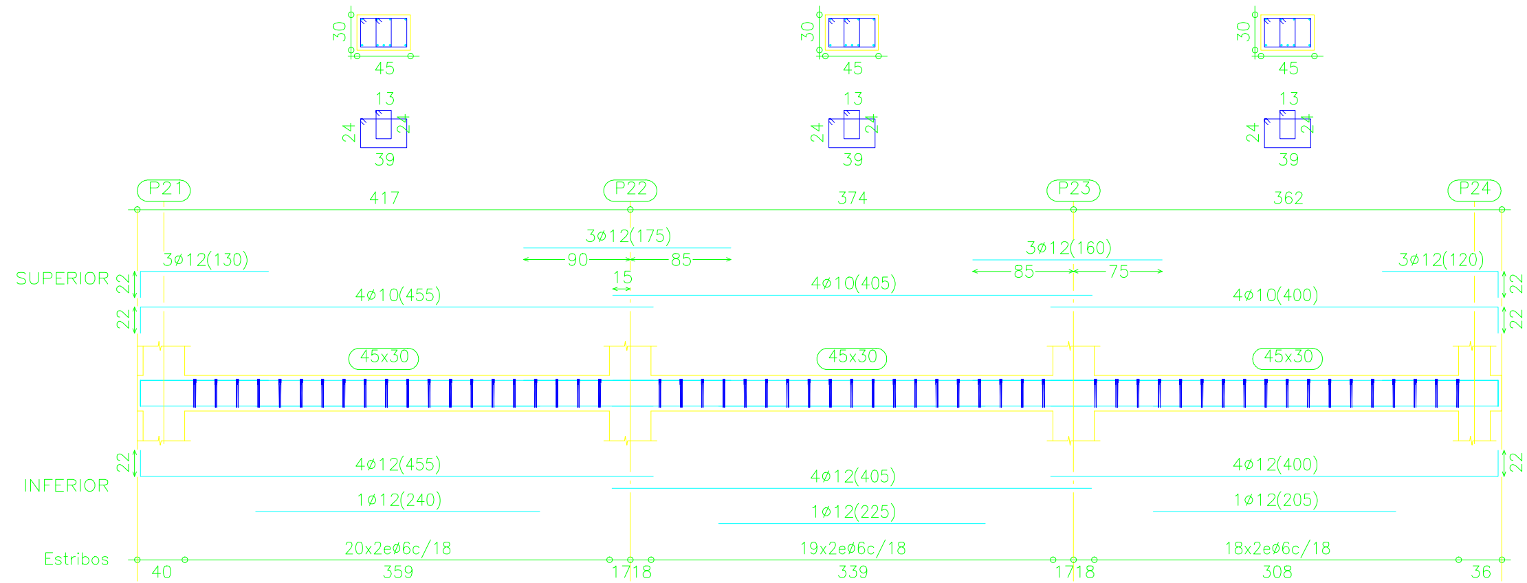
Pórtico 6
