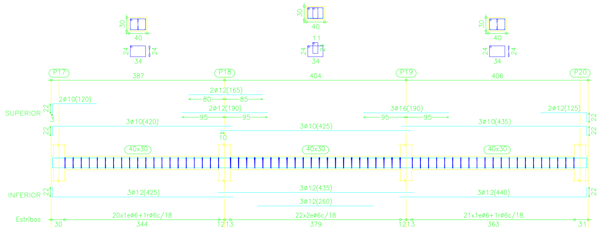
Pórtico 10
