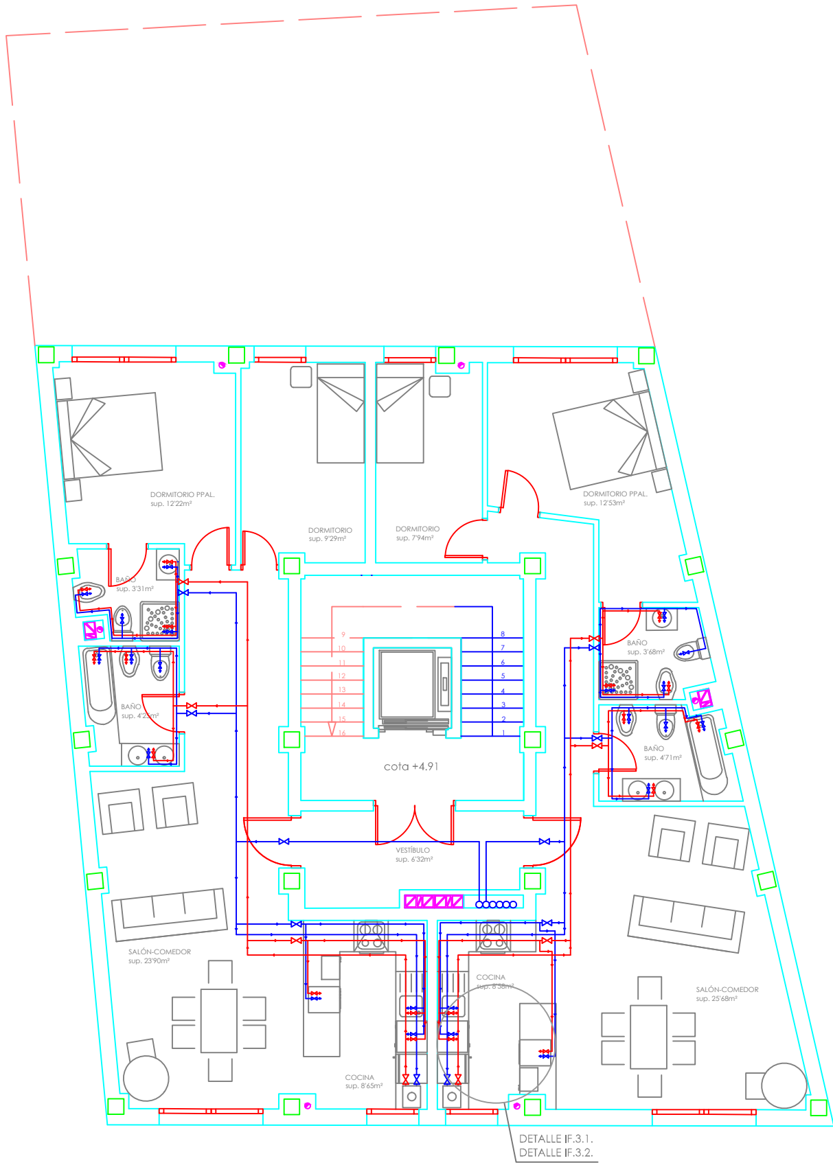
Planta Tipo
