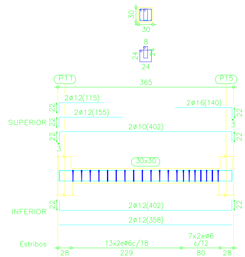
Pórtico 16
