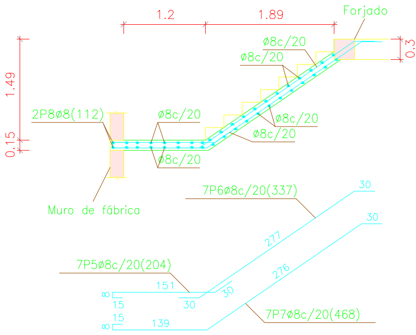
Sección B-B
