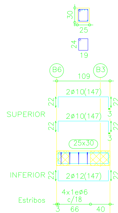
Pórtico 6
