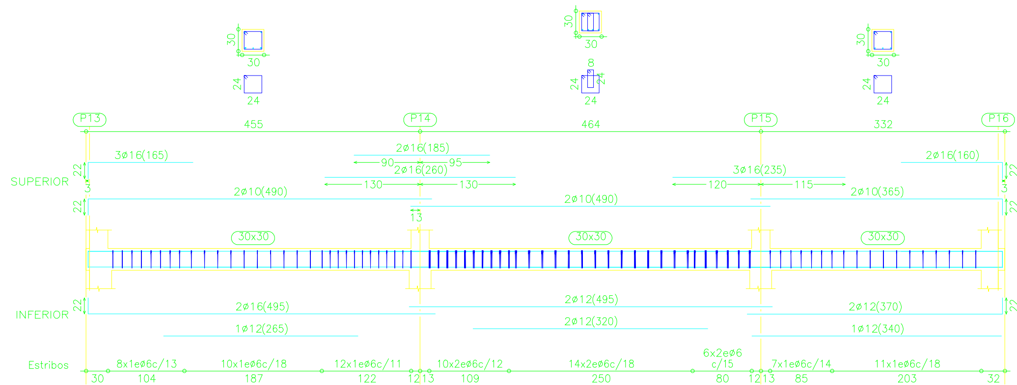
Pórtico 9
