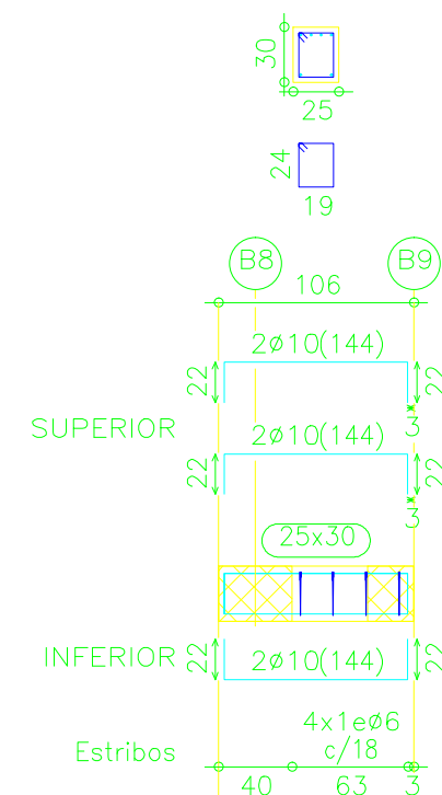
Pórtico 8
