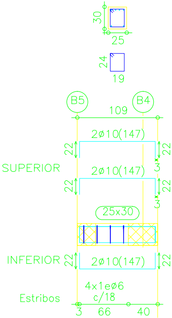
Pórtico 5
