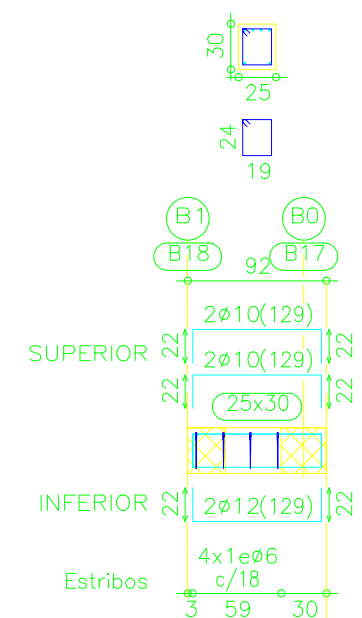
Pórtico 17 Pórtico 20
