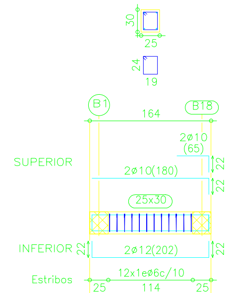
Pórtico 2
