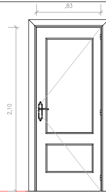
C.I-5: 30 uds. PUERTA BAÑO Y HABITACIONES, DE PASO CIEGA, PRACTICABLE DE 1 HOJA, EN MADERA DE PINO, Y GOMA DE AJUSTE .
