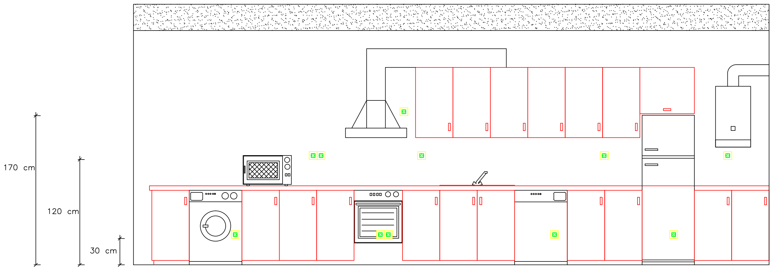
Dotación eléctrica acotada en cocinas
