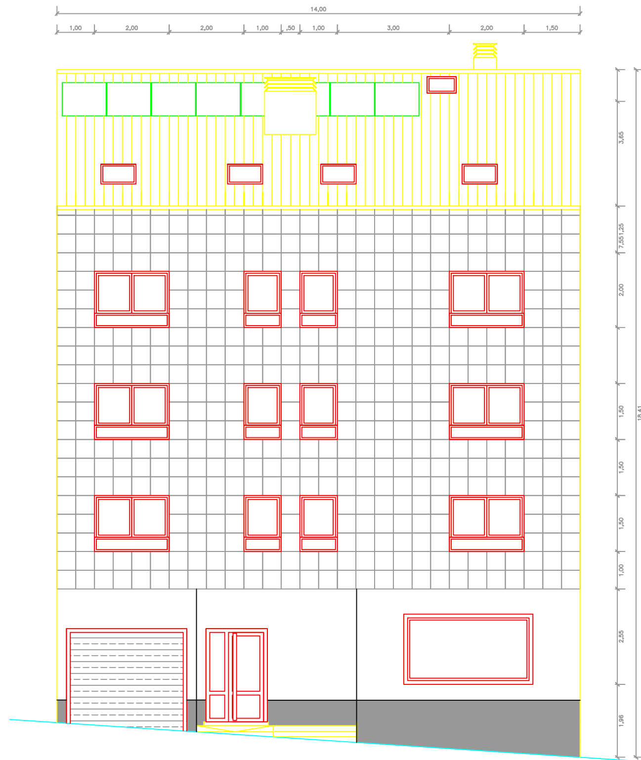
FACHADA DELANTERA
