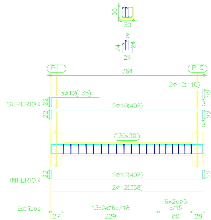
Pórtico 16
