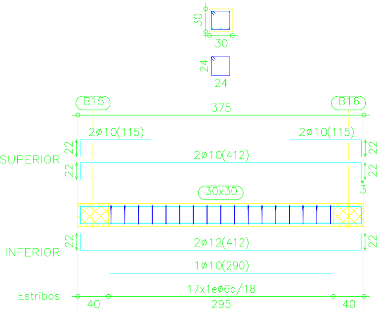
Pórtico 15
