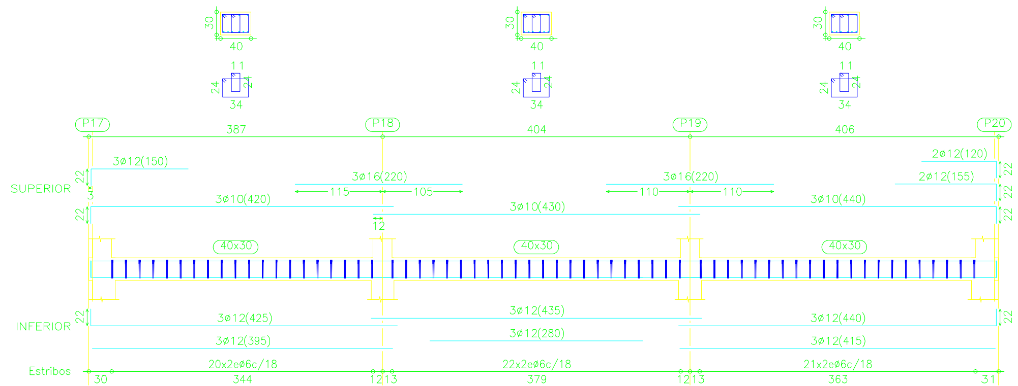
Pórtico 10
