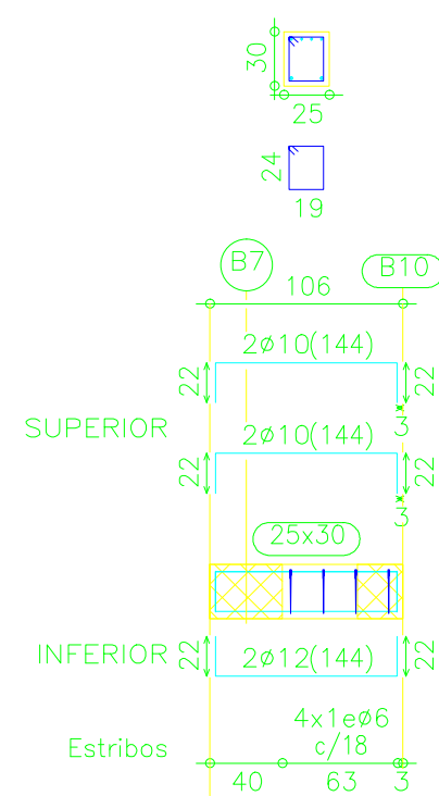
Pórtico 7
