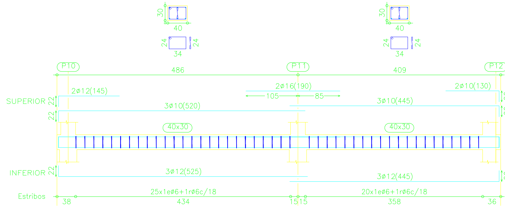
Pórtico 4
