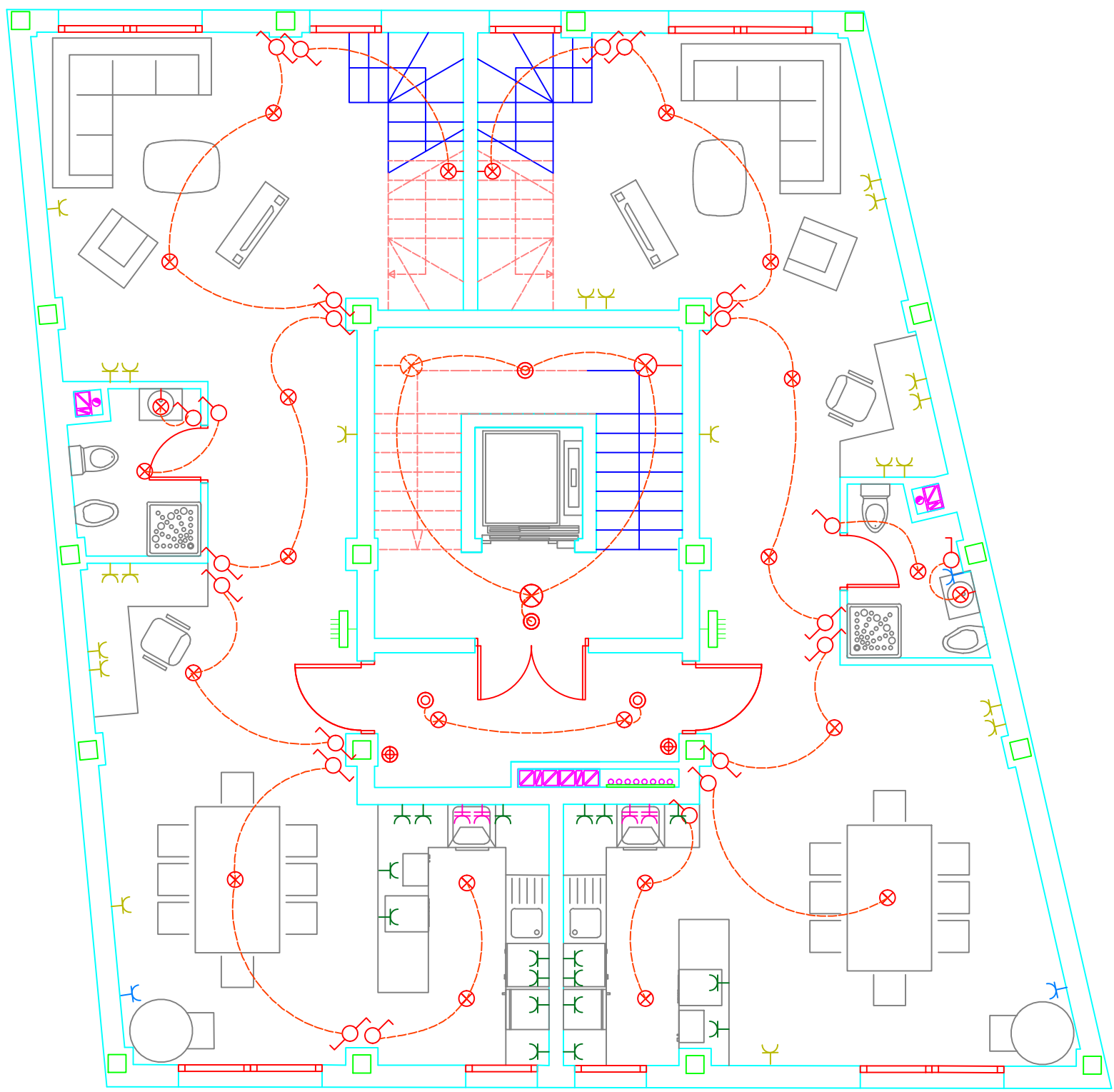
PLANTA 1º DE DÚPLEX
