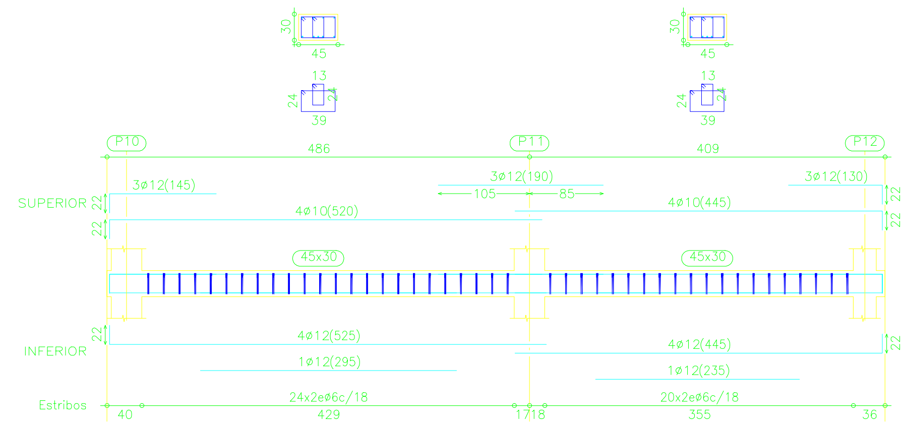
Pórtico 3
