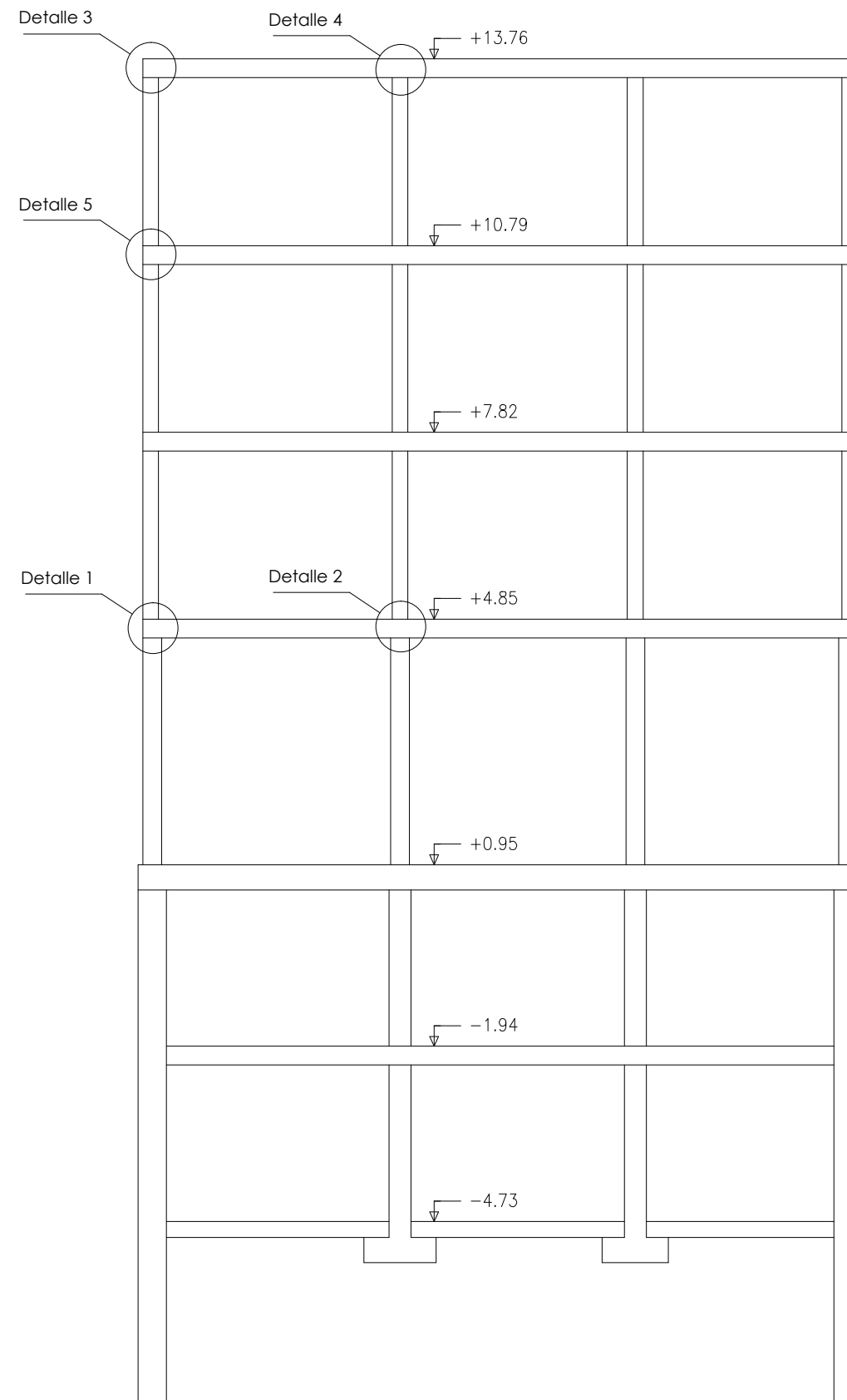
ALINEACIÓN 6
