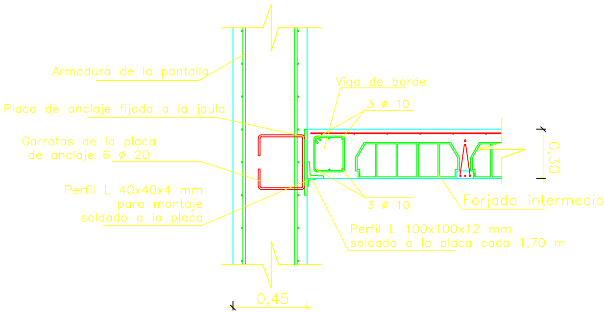
Detalle 7: Encuentro de forjado intermedio paralelo con pantalla
