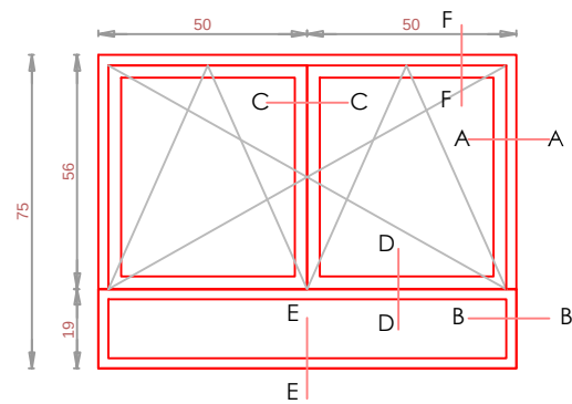
C-1 VENTANA OSCIOBATIENTE DE PVC DE DOS HOJAS CON MONTANTE INFERIOR FIJO
