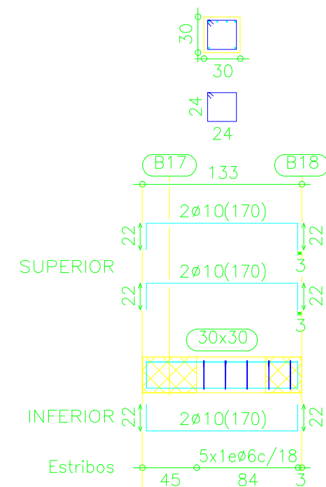
Pórtico 7
