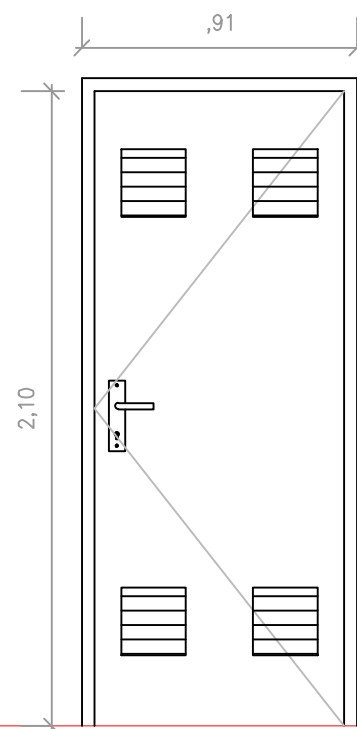
C.I-1 : 13 uds. PUERTA DE TRASTEROS Y CUARTOS DE INSTALACIONES METÁLICA PRACTICABLE 1 HOJA, CON REJILLAS DE VENTILACIÓN. LACADA AL HORNO CON RAL 9006, CON CERRADURA DE COMPAÑIA
