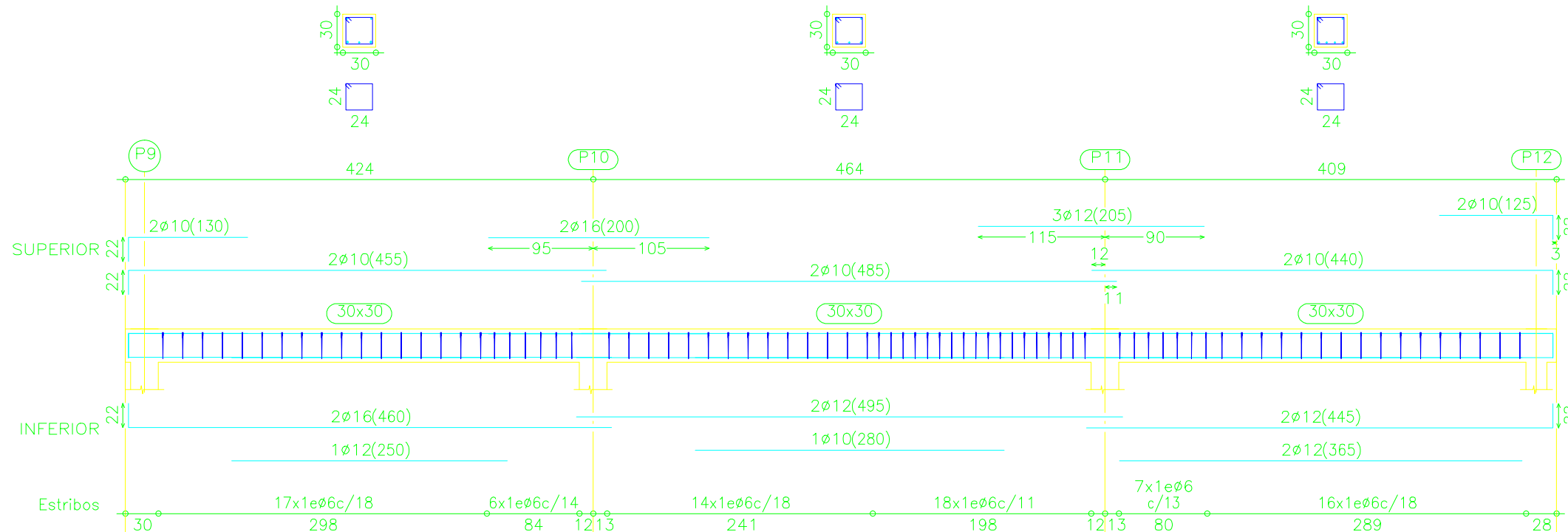
Pórtico 6
