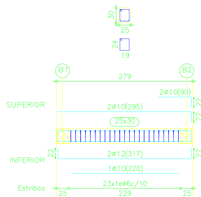
Pórtico 2
