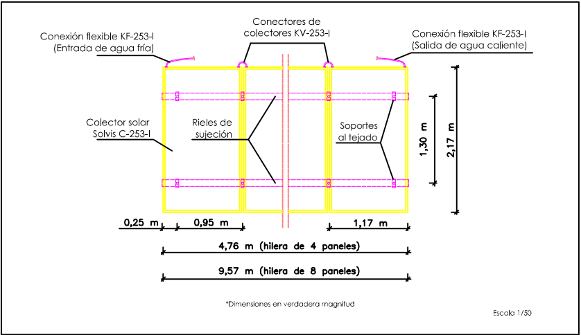
Montaje de colectores solares en serie sobre cubierta inclinada
