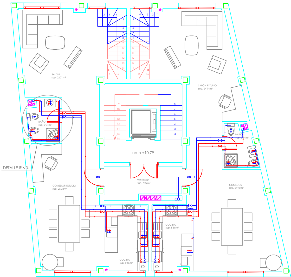
Planta Tercera 1Ü Nivel D1/plex
