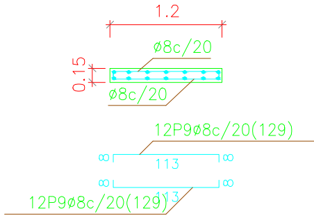
Sección D-D
