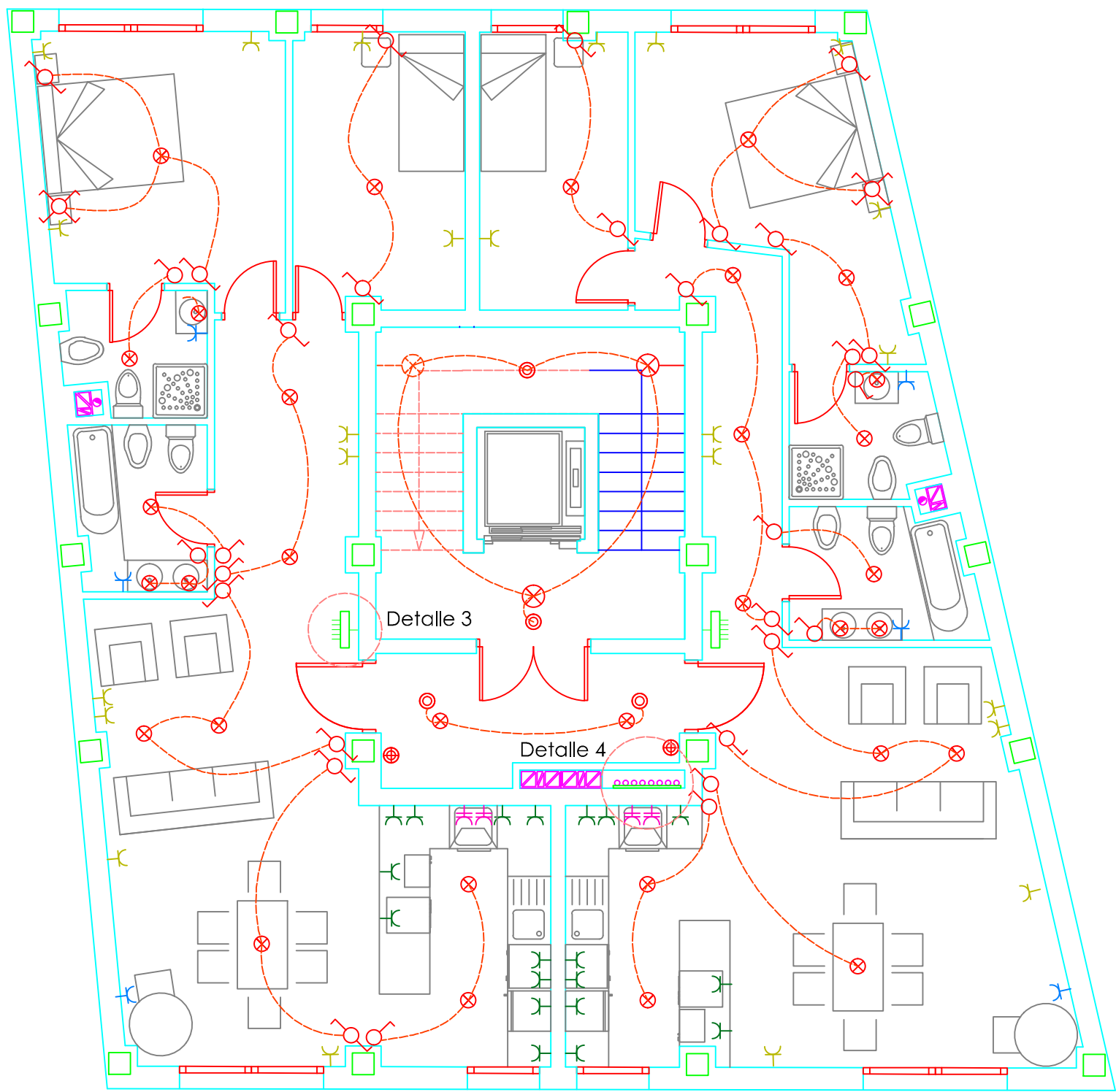
PLANTA 1º Y 2º
