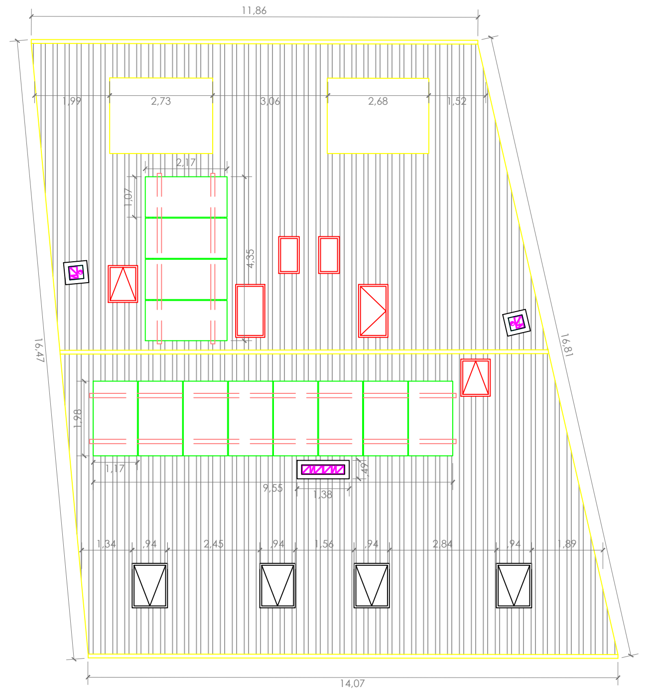
Planta Cubierta
