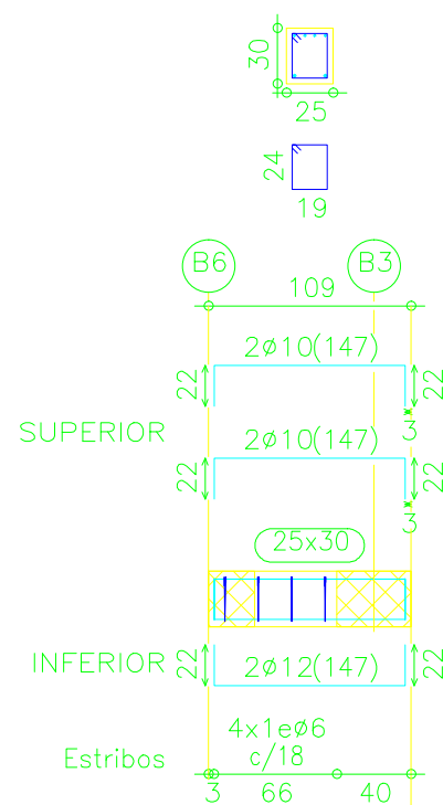
Pórtico 6
