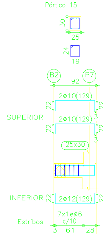
Pórtico 15
