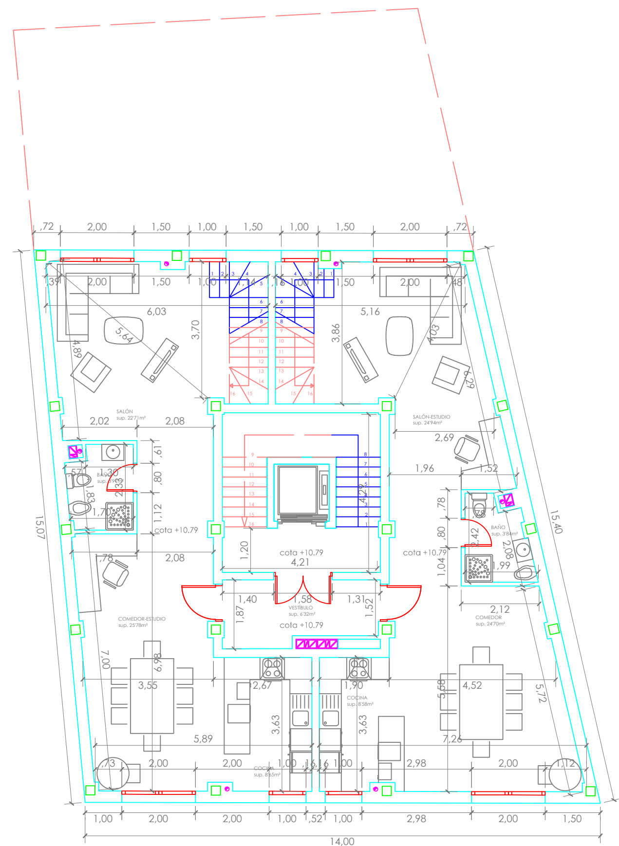
Planta Tercera 1º Nivel Dúplex
