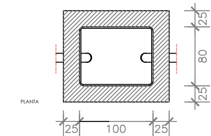
ARQUETA SEPARADORA DE GRASAS E: 1/50
