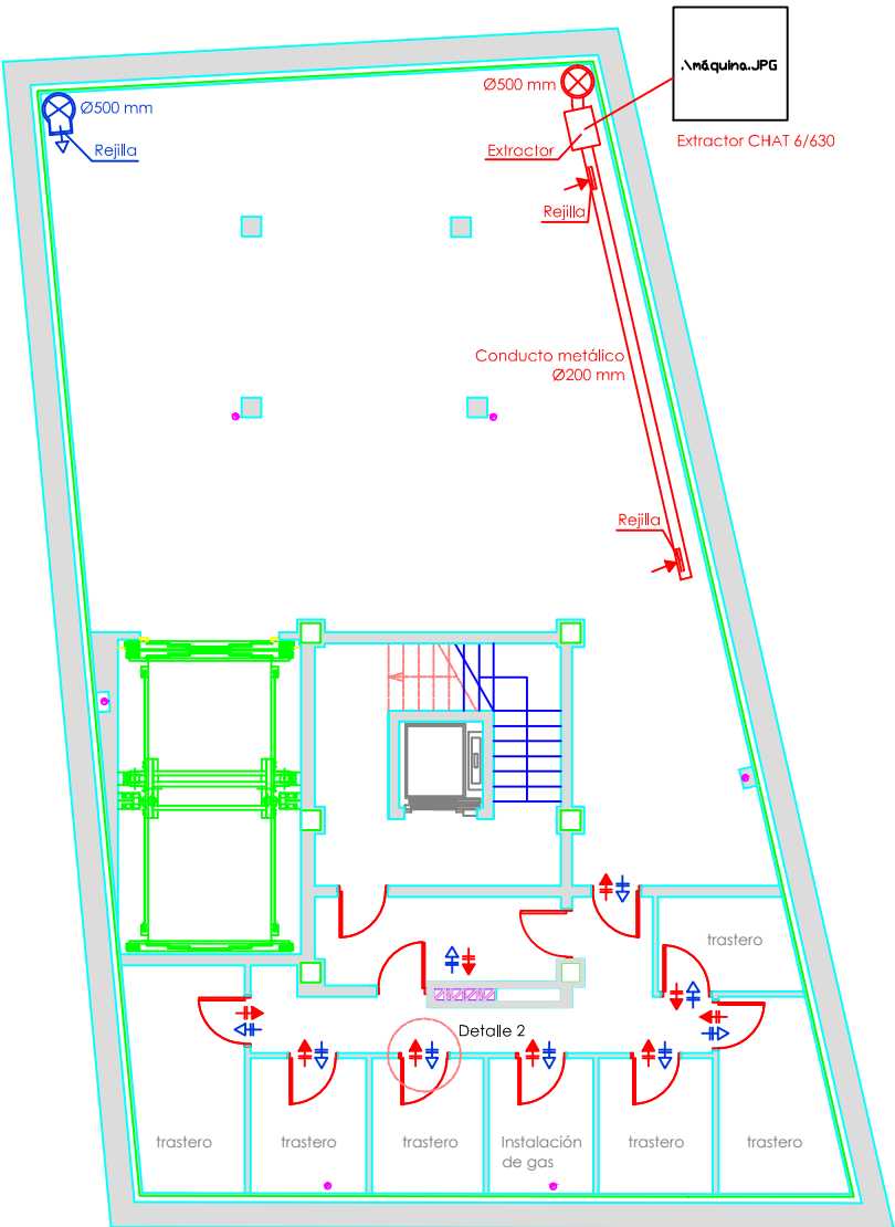
PLANTA SÓTANO 1
