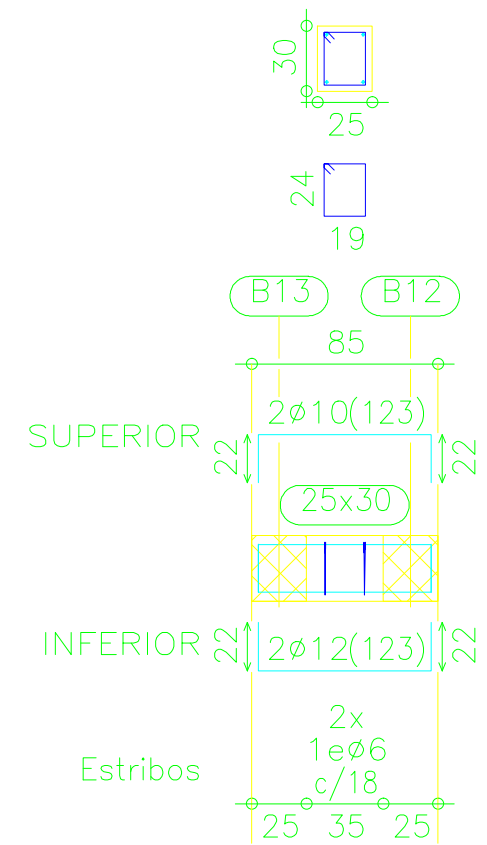
Pórtico 21
