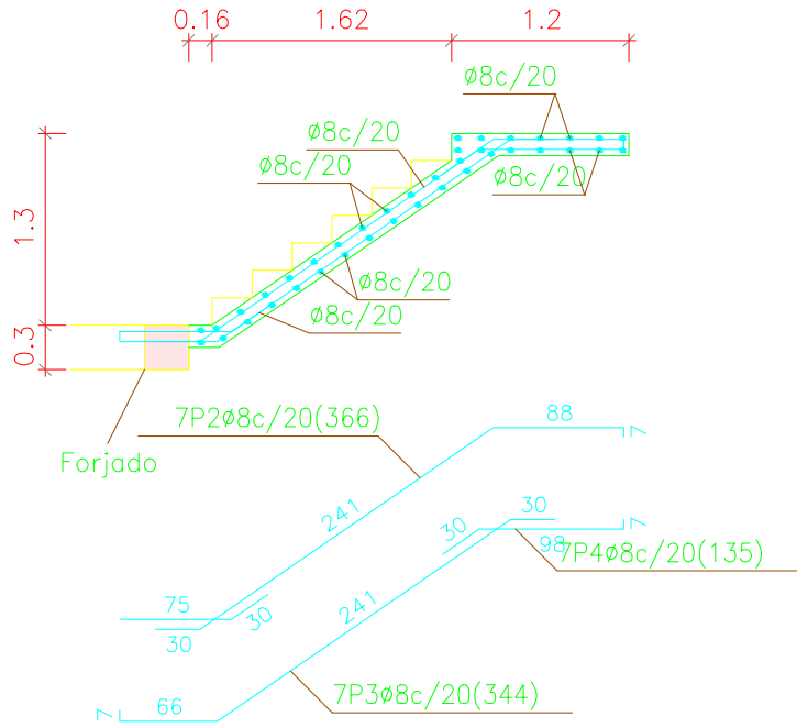
Sección A-A
