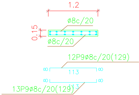
Sección C-C
