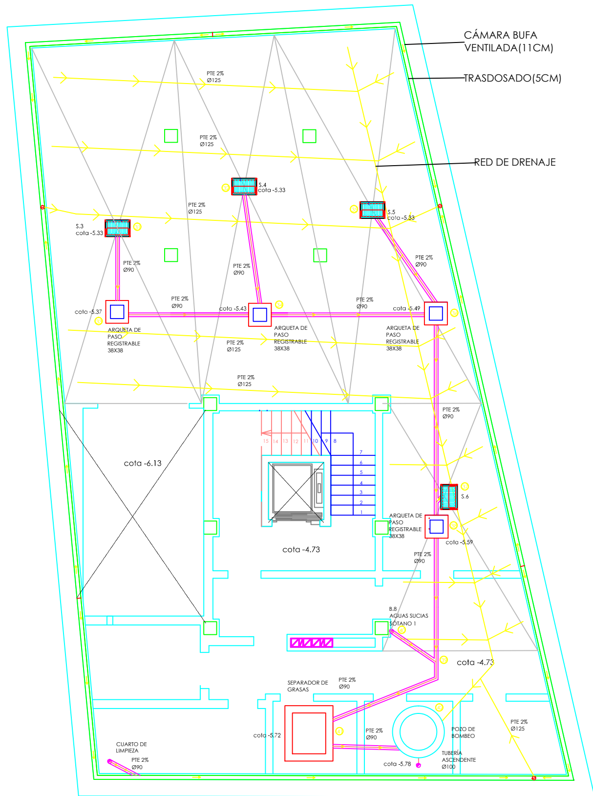
Planta Sótano 2º
