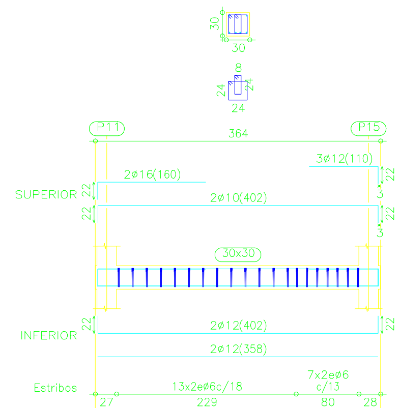
Pórtico 16
