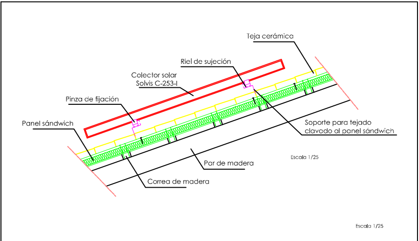
Detalle de la sujeción de los paneles a la cubierta
